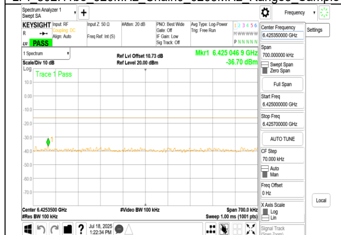
LPI 802.11be 320MHz Chain1 6105MHz Range2
