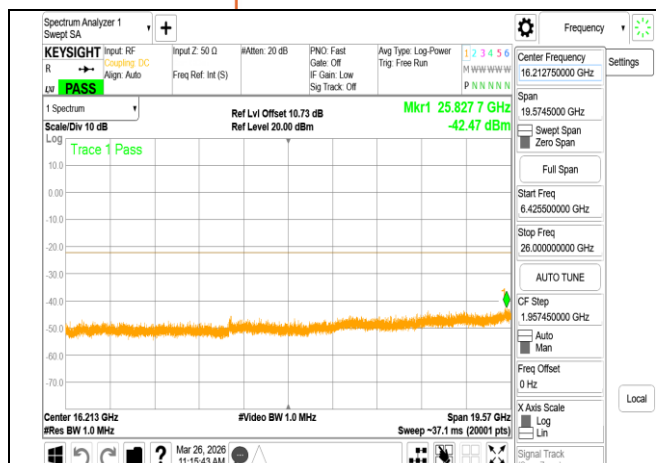
VLP 802.11n 20MHz Chain1 5955MHz Range3
