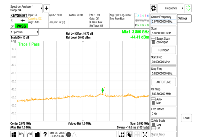
VLP 802.11n 20MHz Chain1 6175MHz Range1
