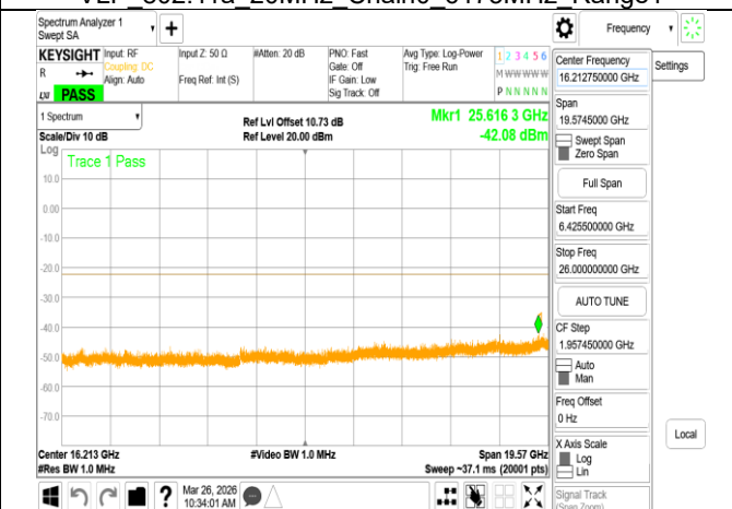
VLP_802.11a_20MHz_Chain0_6175MHz_Range3
