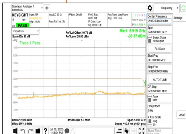
LPI 802.11be 320MHz Chain1 6265MHz Range1
