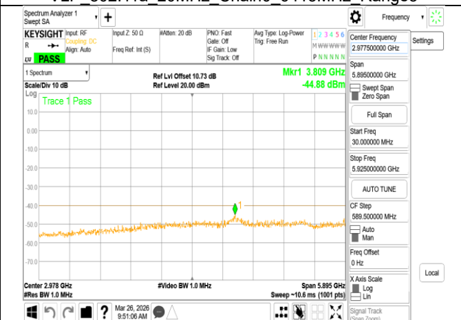
VLP_802.11a_20MHz_Chain1_5955MHz_Range1
