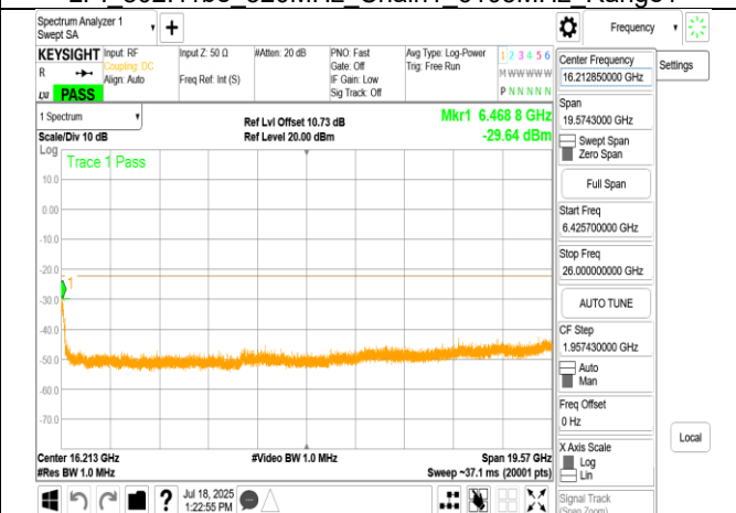
LPI 802.11be 320MHz Chain1 6105MHz Range3
