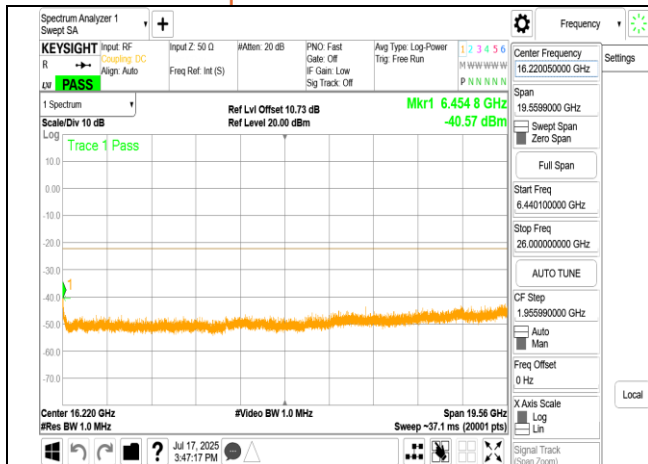
LPI 802.11be 40MHz Chain0 6405MHz Range3
