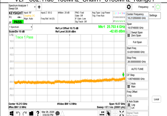
VLP 802.11ac 160MHz Chain1 6185MHz Range3
