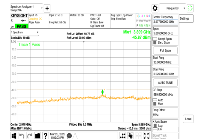
VLP 802.11ax 20MHz Chain0 5955MHz Range1
