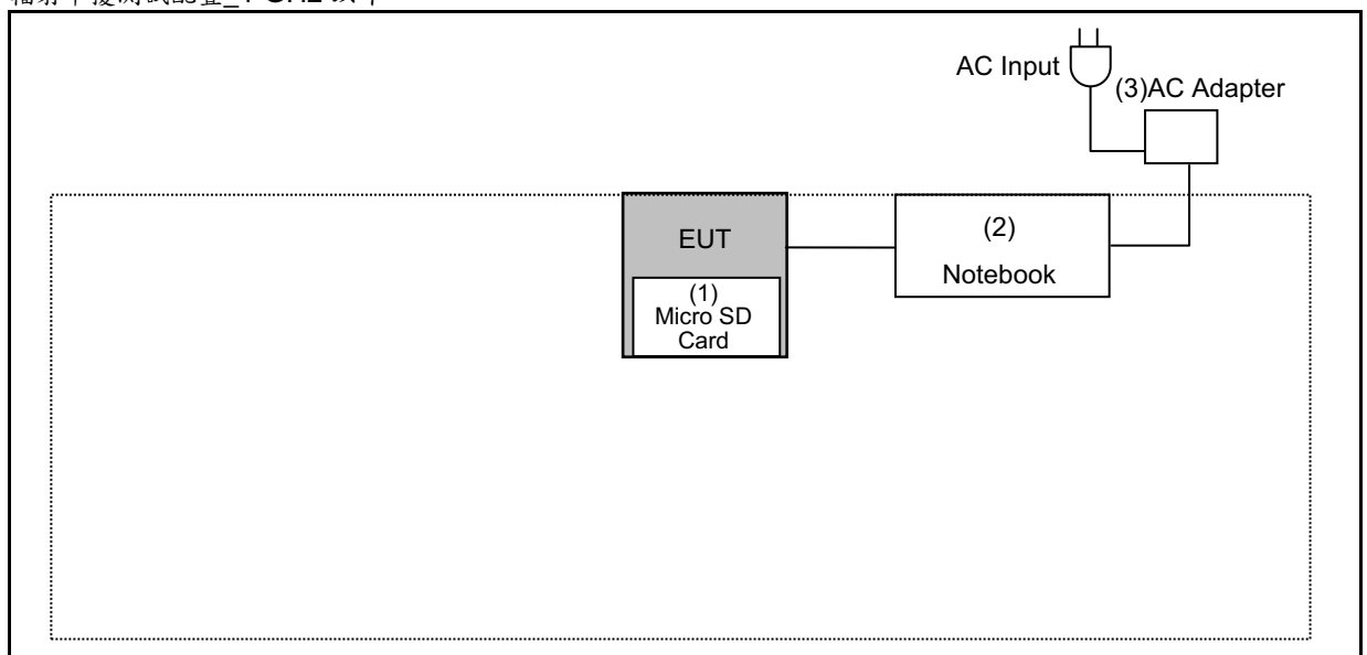
輻射干擾測試配置_1 GHz 以下
