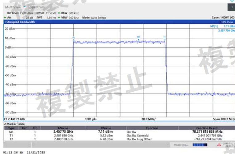
NTVN-2DH5-Ant1-Hop-PASS
