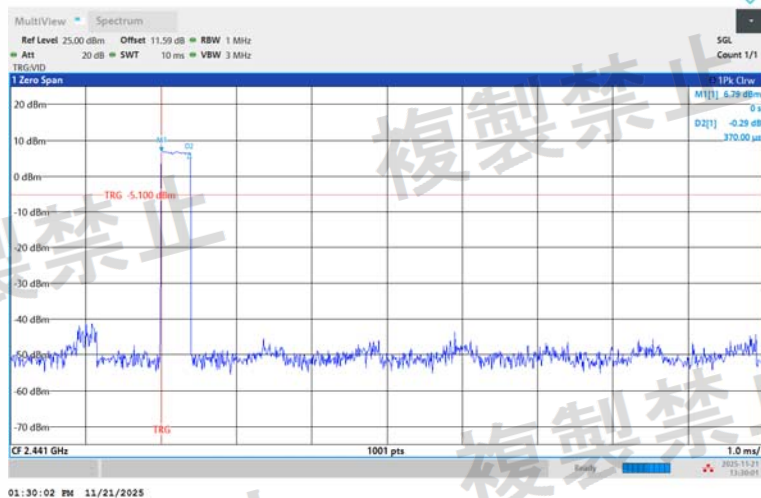
NTNV-2DH1-Ant1-Hop-PASS
