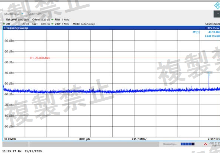
NTNV-2DH5-Ant1-2441-30~2387-PASS
