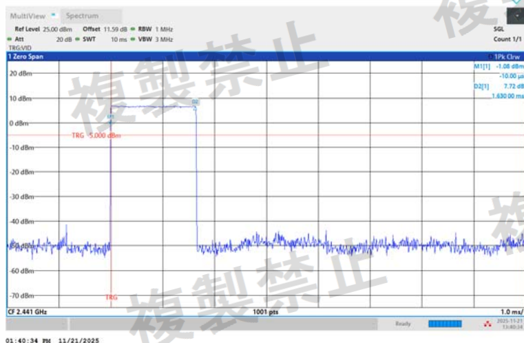
NTNV-2DH3-Ant1-Hop-PASS
