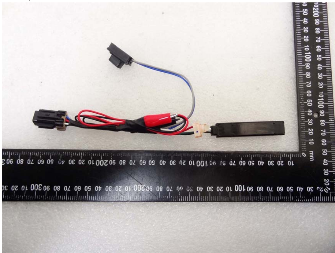
EUT-20. AST Antenna
