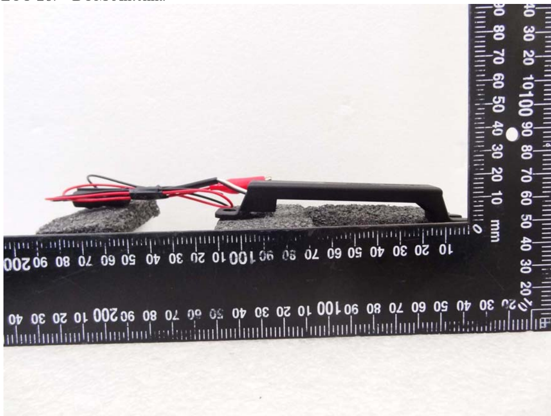
EUT-28. BUM Antenna
