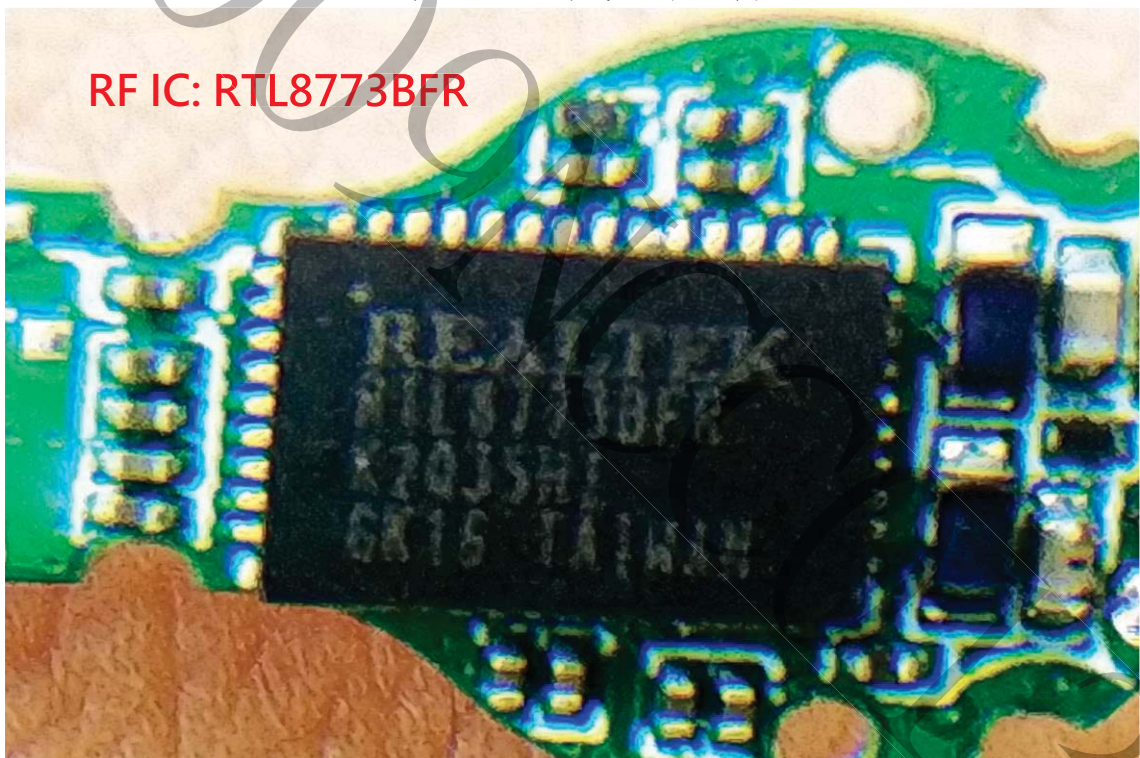
16) 模組特寫照(右耳)
