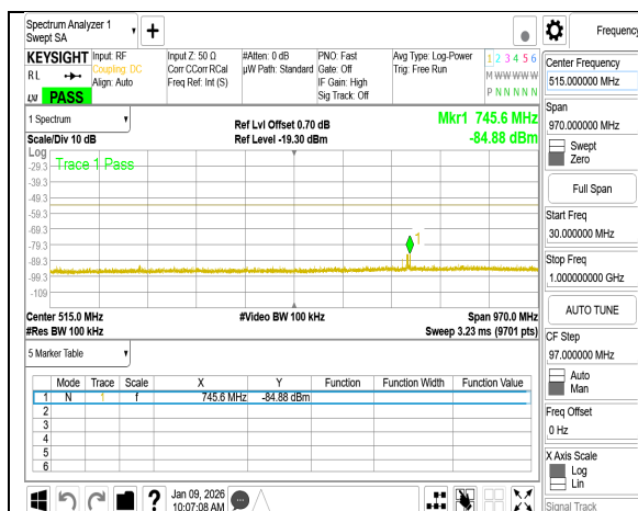
RX Below 1GHz BLE 1M 2402MHz
