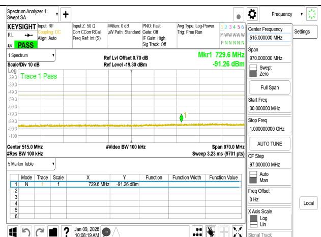
RX Below 1GHz BLE 1M 2480MHz
