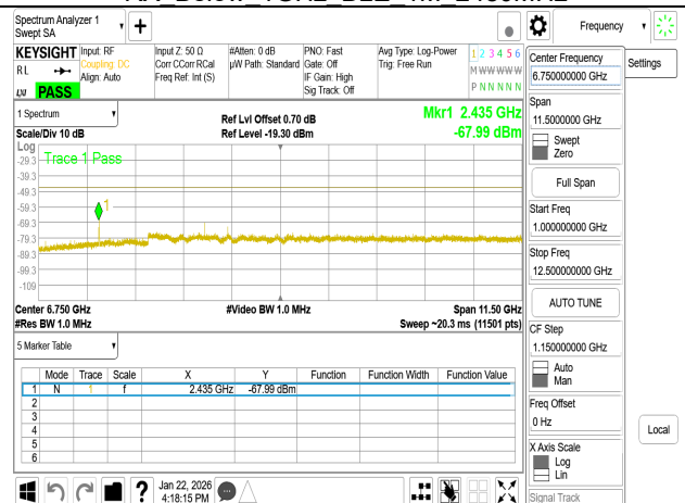
RX Above 1GHz BLE 1M 2480MHz
