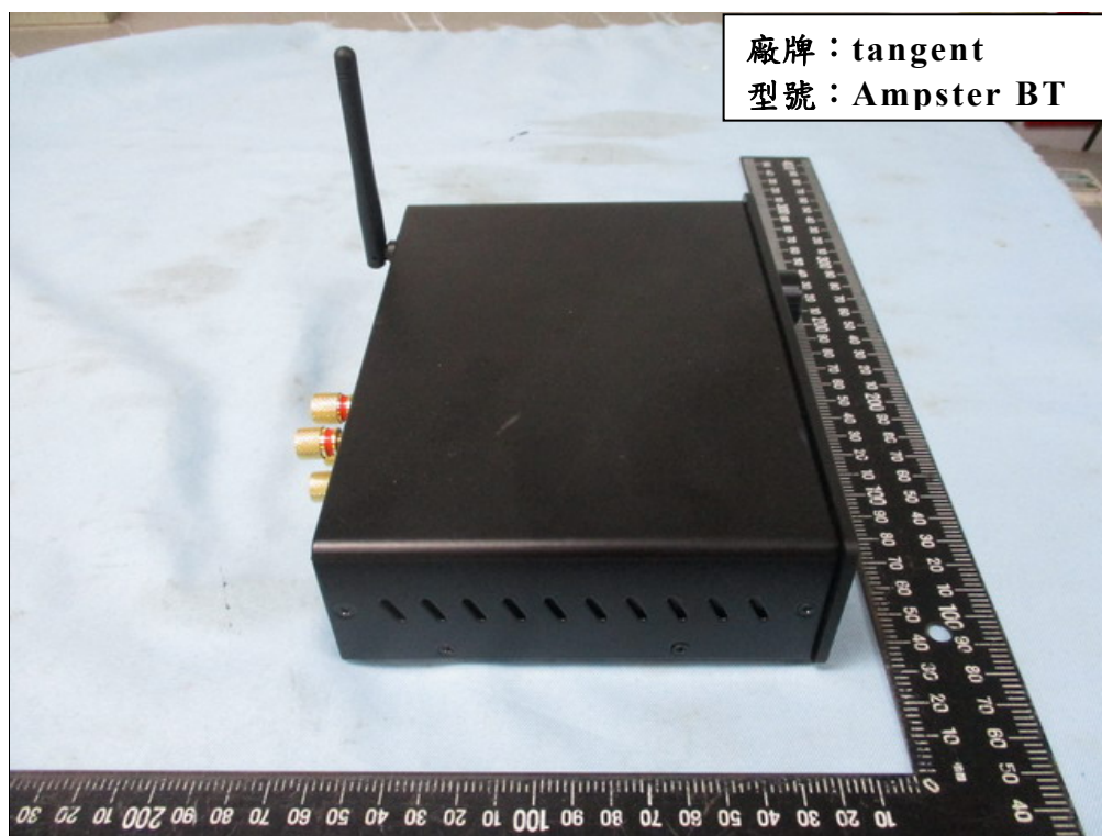
產品外觀照
