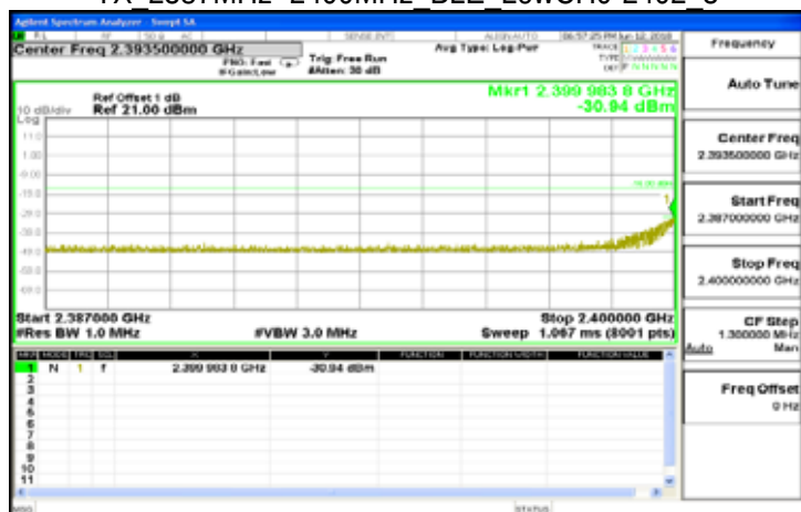
TX 2387MHz~2400MHz_BLE_LowCH0-2402_3
