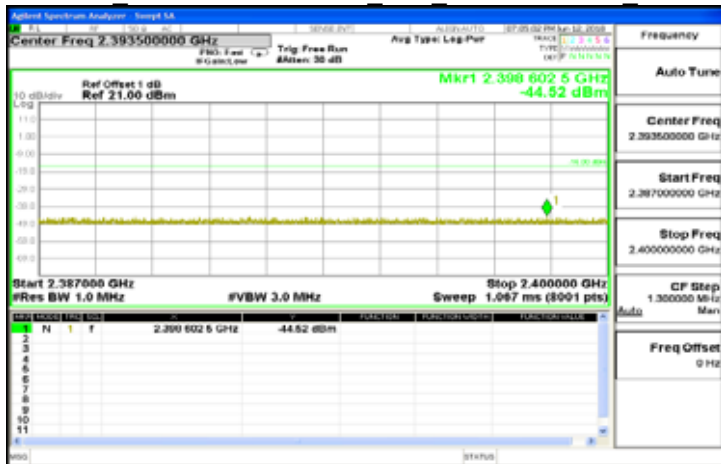
TX 2387MHz~2400MHz BLE MidCH20-2442 3
