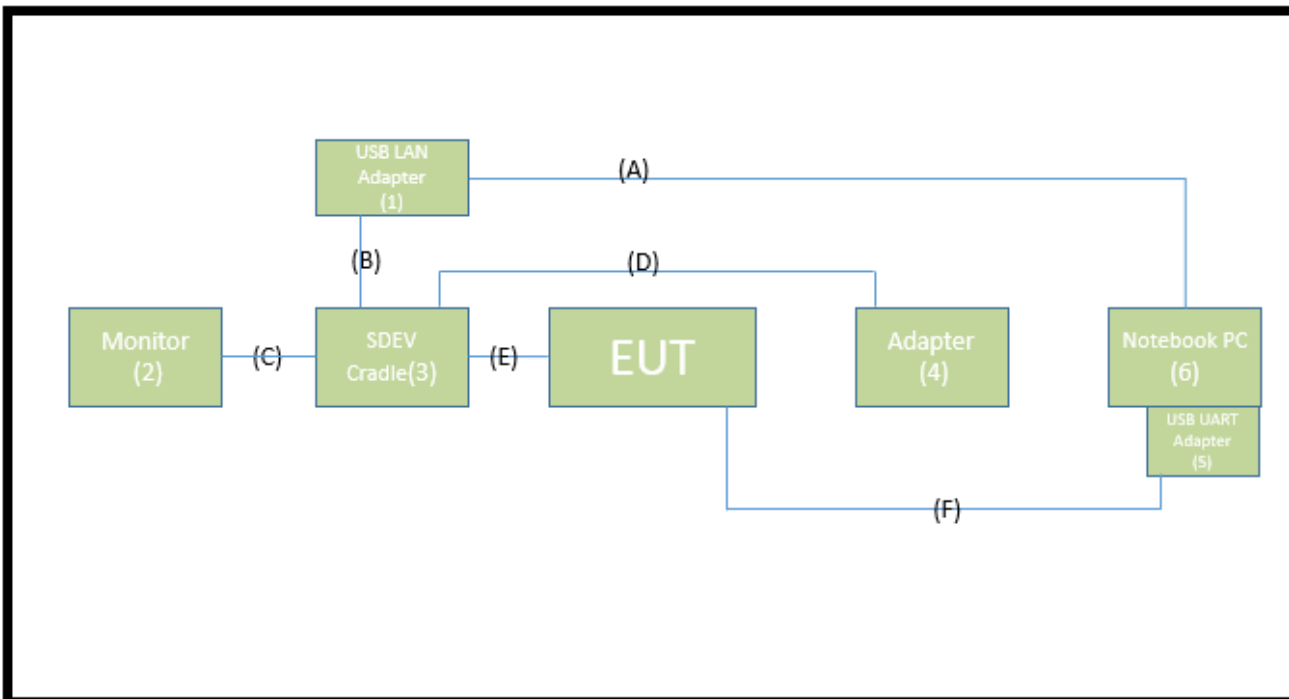
待測物測試配置圖 (Mode1~Mode3)
