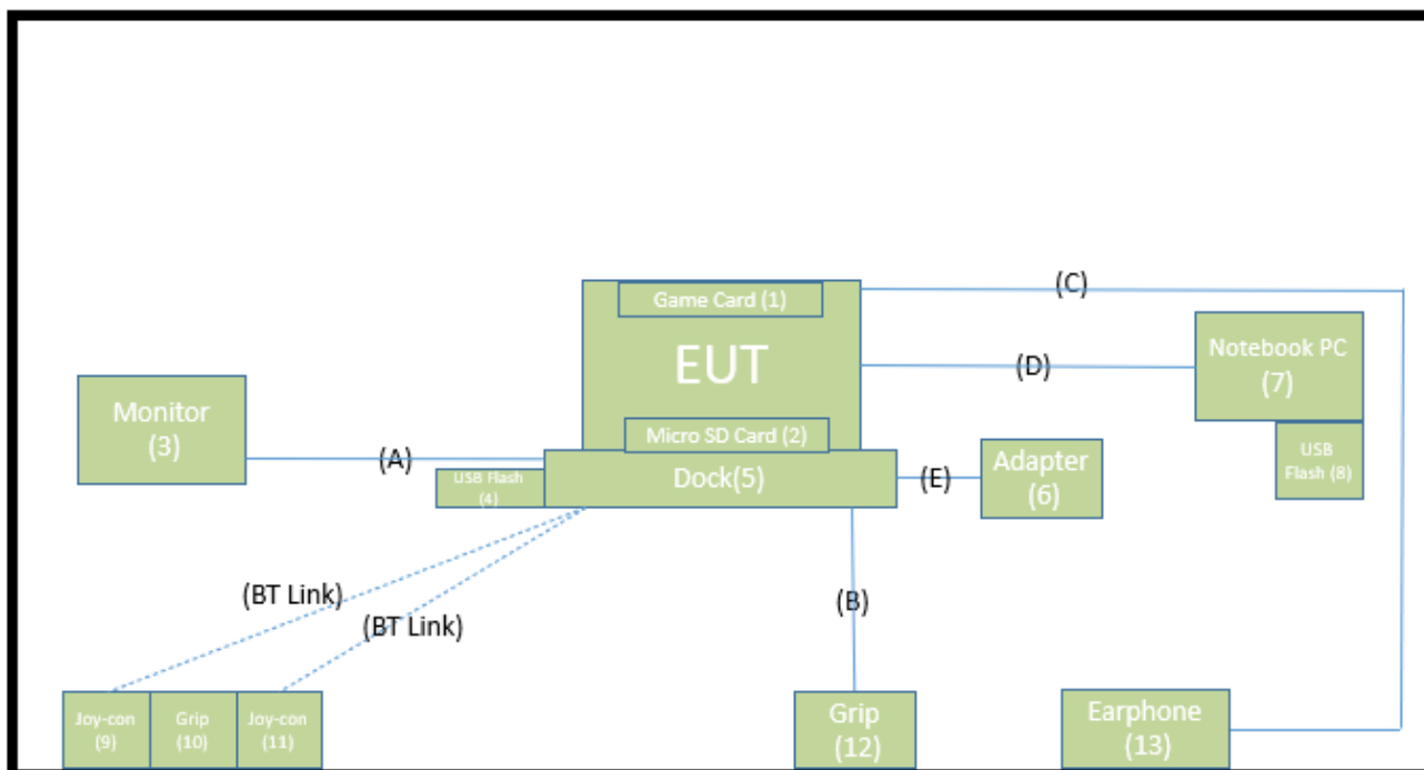
待測物測試配置圖 (Normal Mode / Mode4)
