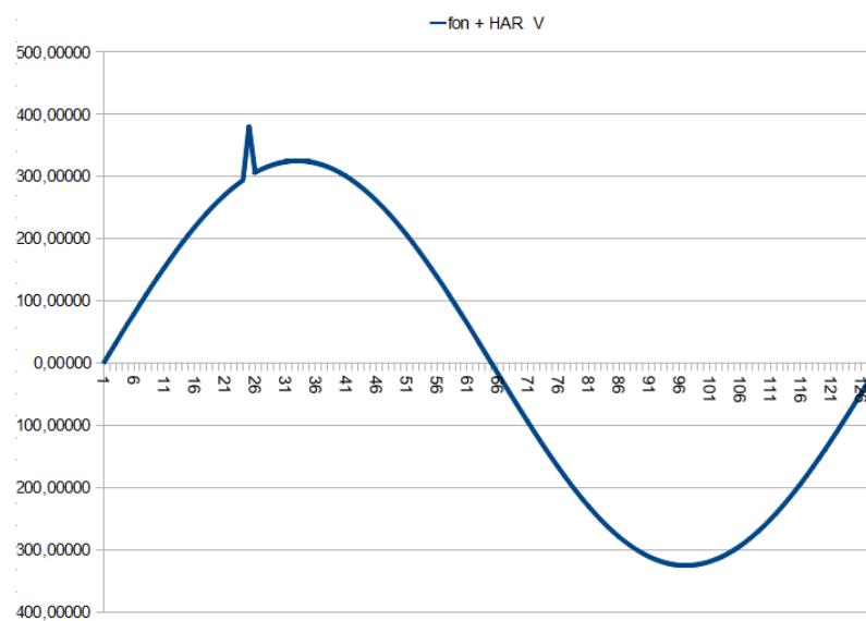
Figure 29: Transitoires détectés avec un coefficient de distorsion de 5.0.
