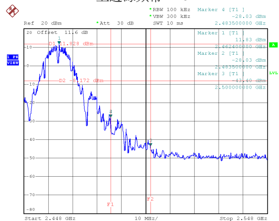
上邊緣頻帶-2462 MHz
