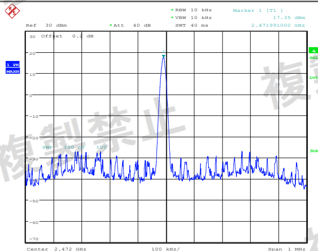
NTVN_11G_Ant1_2472
