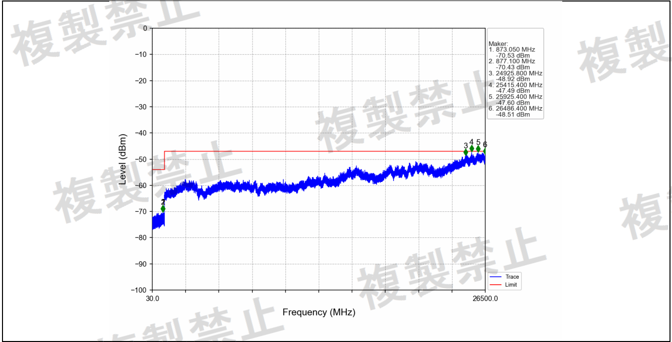
802.11be(EHT160)_MCH_5250MHz_SU / _MIMO_NTNV
