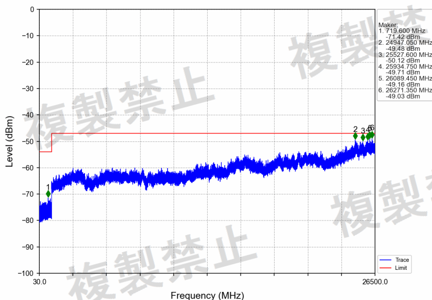
802.11be(EHT20) HCH 5240MHz SU / MIMO NTNv
