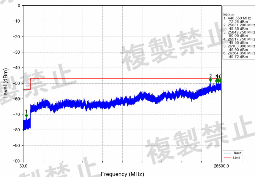
802.11be(EHT20) HCH 5240MHz SU / Ant2 NTNv
