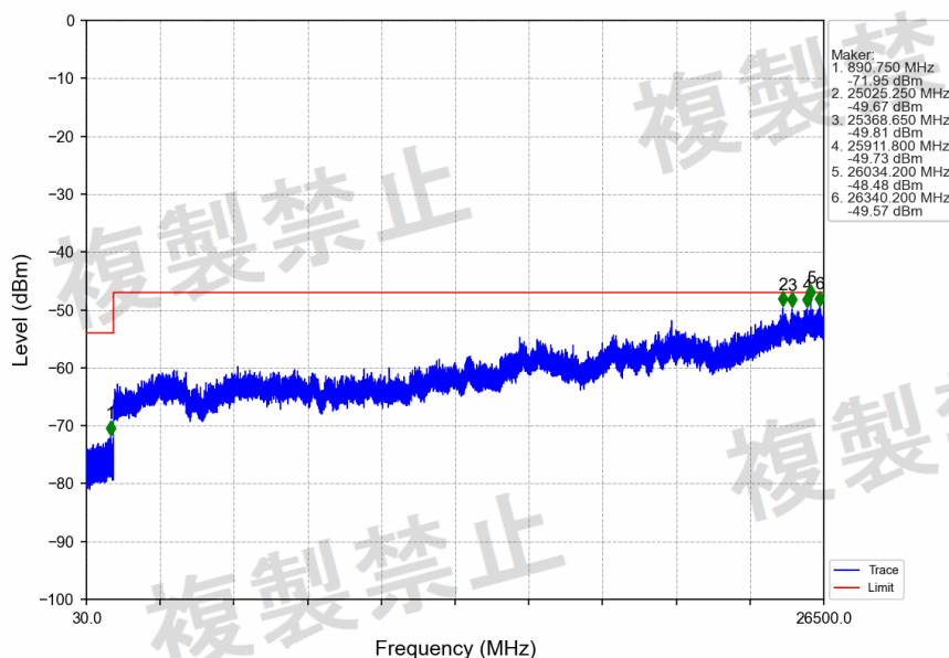
802.11be(EHT40) HCH 5310MHz SU / MIMO NTNv
