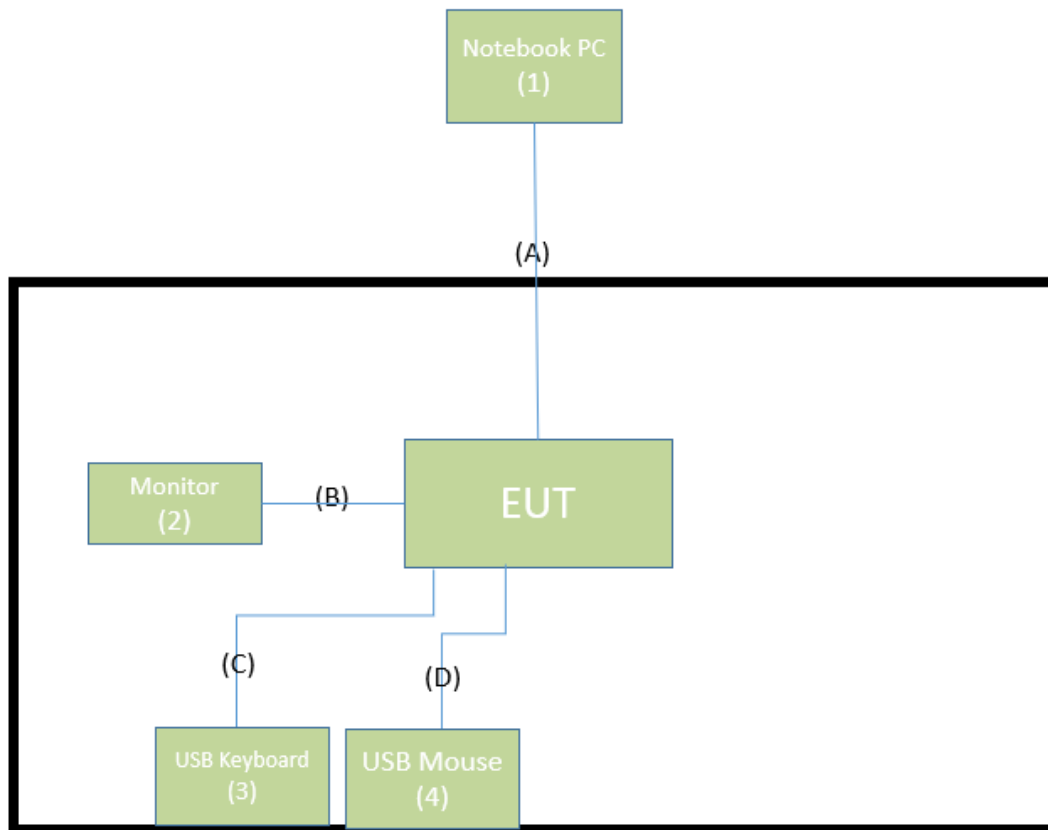
待測物測試配置圖
