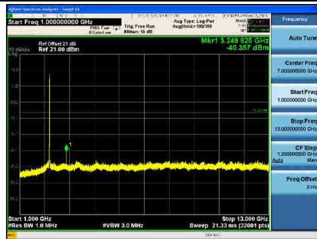
802.11 b CH11 (2462MHz) Ant 0
