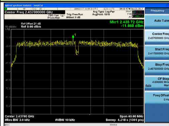
802.11 n-40M CH 06 (2437MHz) Ant 0
