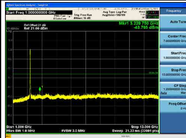
802.11 n40 CH06 (2437MHz) Ant 0
