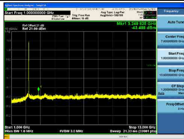
802.11 g CH11 (2462MHz) Ant 0
