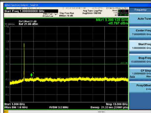
802.11 n40 CH09 (2452MHz) Ant 1
