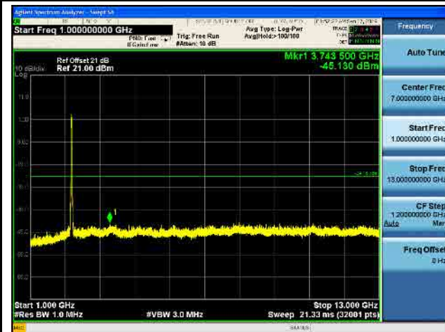
802.11 n40 CH06 (2437MHz) Ant 1
