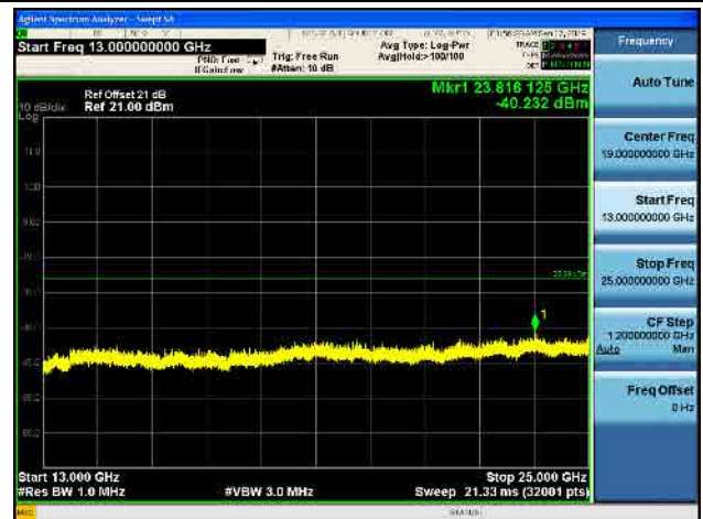
802.11 n40 CH06 (2437MHz) Ant 0
