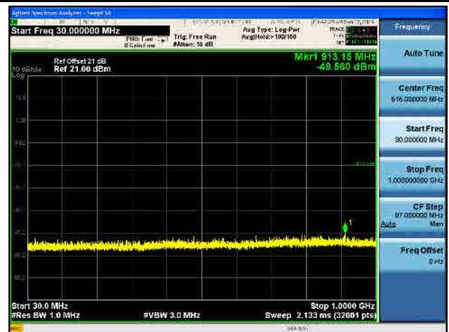
802.11 n20 CH06 (2437MHz) Ant 0
