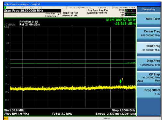
802.11 n40 CH03 (2422MHz) Ant 1
