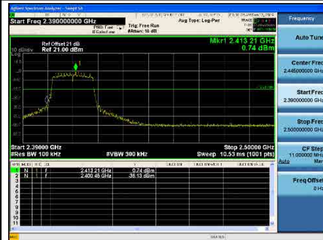
802.11 n20 CH01 (2412MHz) Ant 0
