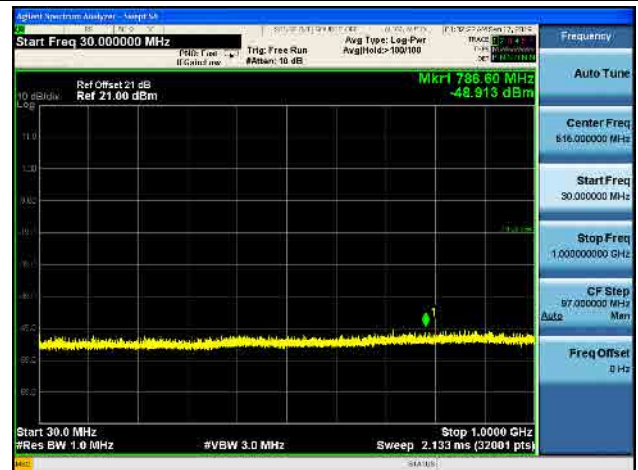
802.11 n20 CH01 (2412MHz) Ant 0
