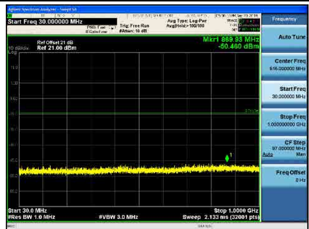
802.11 n40 CH06 (2437MHz) Ant 1
