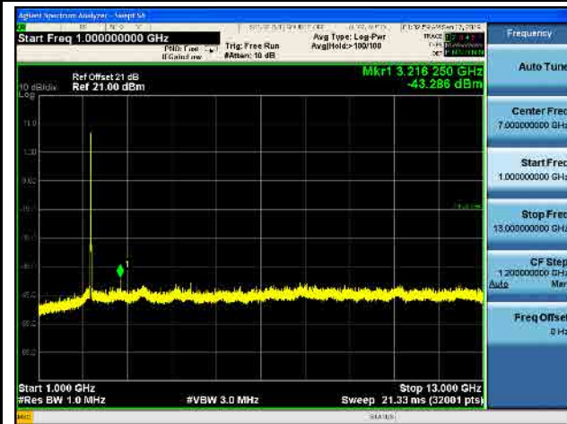
802.11 n20 CH06 (2437MHz) Ant 0
