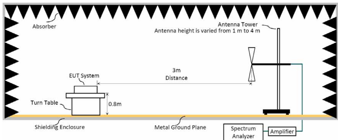
圖 2: 量測場地(No. 4 3m Chamber)量測頻率高於 1GHz 之測試配置
