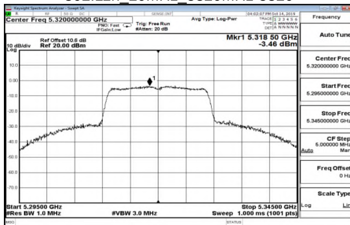
802.11n 20MHz 5320MHz-5320
