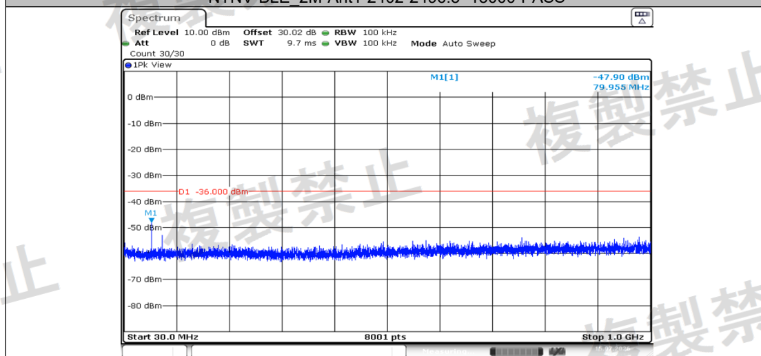
NTNV-BLE_2M-Ant1-2440-30~1000-PASS
