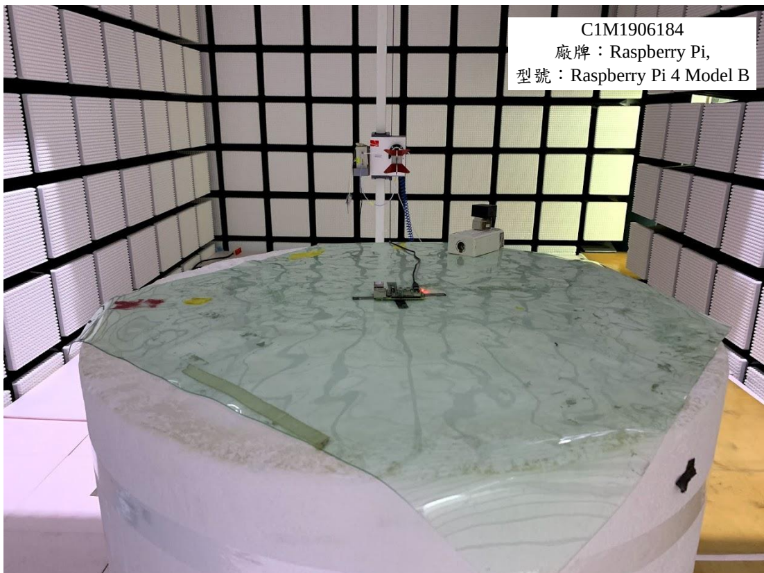
2.2 量測頻率高於 1GHz 之測試 發射/接收模式 單機-平放
