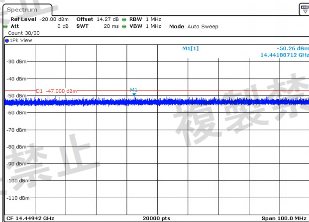
NTNV-11AC20-Ant1-5500-1000~26000-PASS
