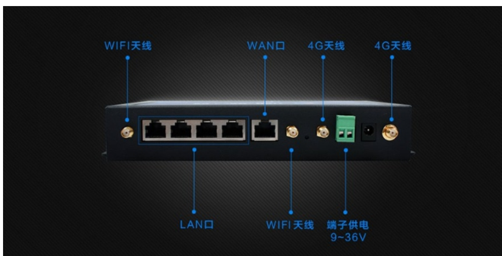
图 1 G800V2 接口图
