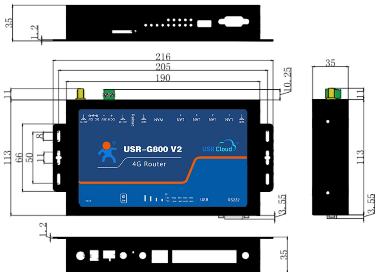
图 2 G800V2 外观尺寸图
