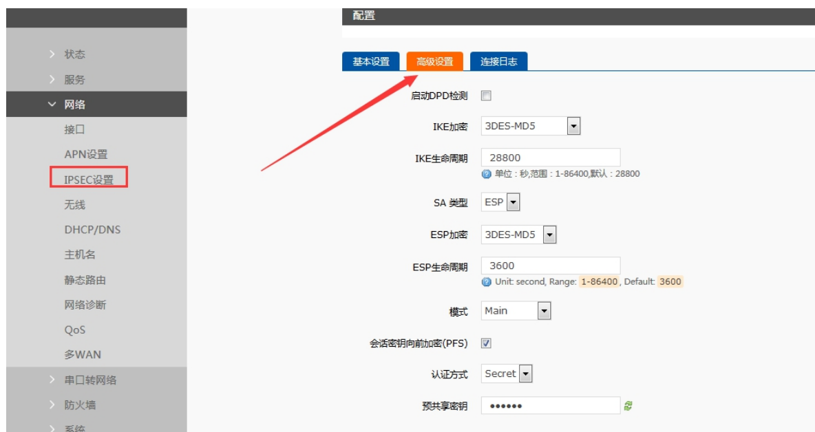
图 78 IPsec 测试 3
