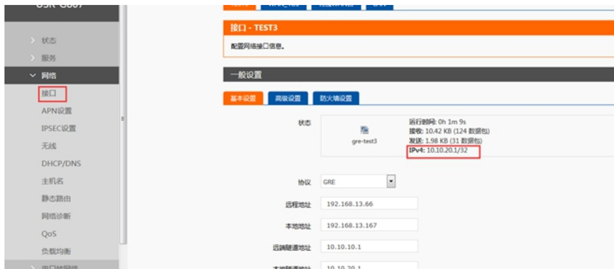
图 95 GRE 测试 2
