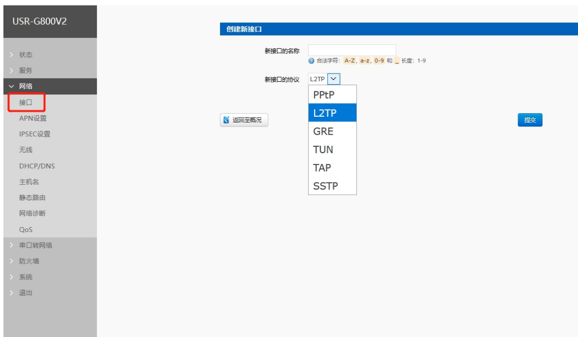
图 71 创建接口
