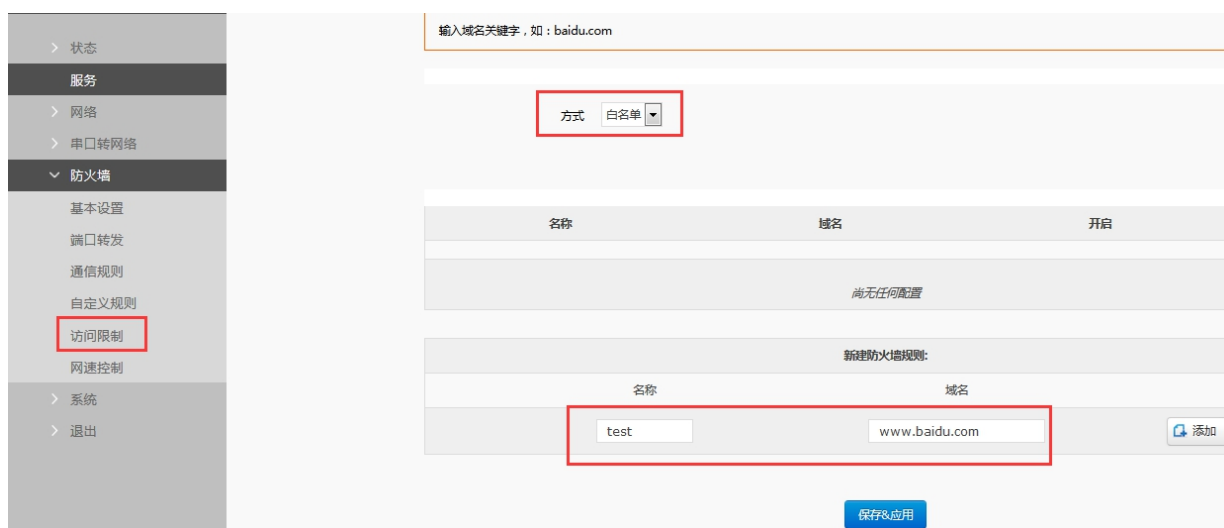
图 128 域名白名单
