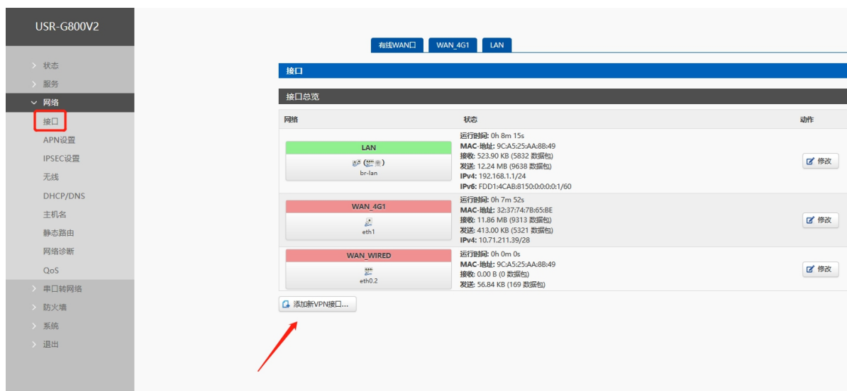
图 85 创建接口
