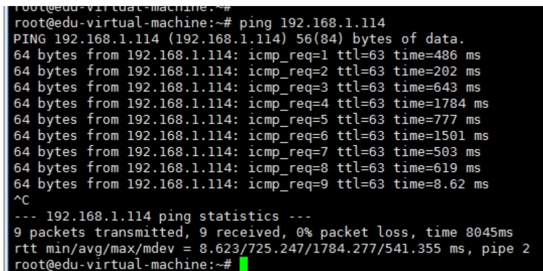
图 80 IPSec 测试 5
