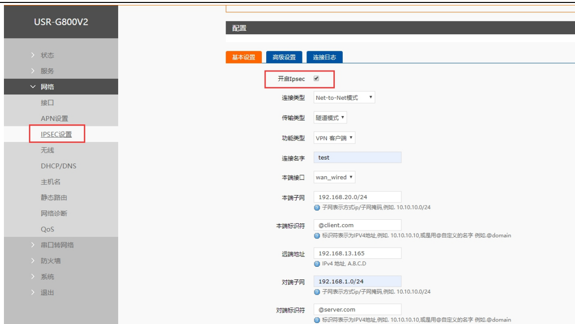
图 81 IPsec 测试 6
