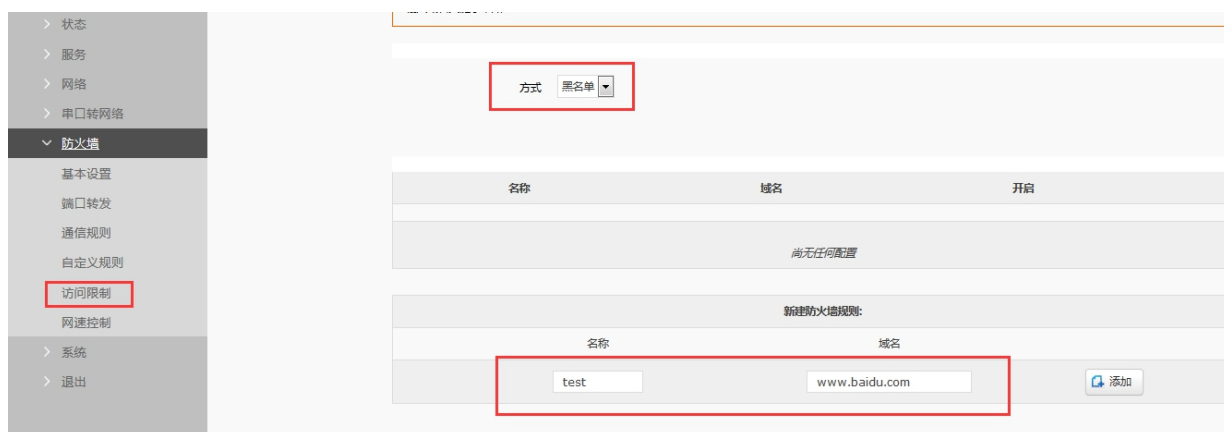
图 127 域名黑名单
