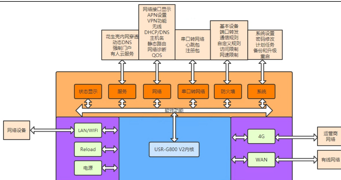
图 3 功能框图
