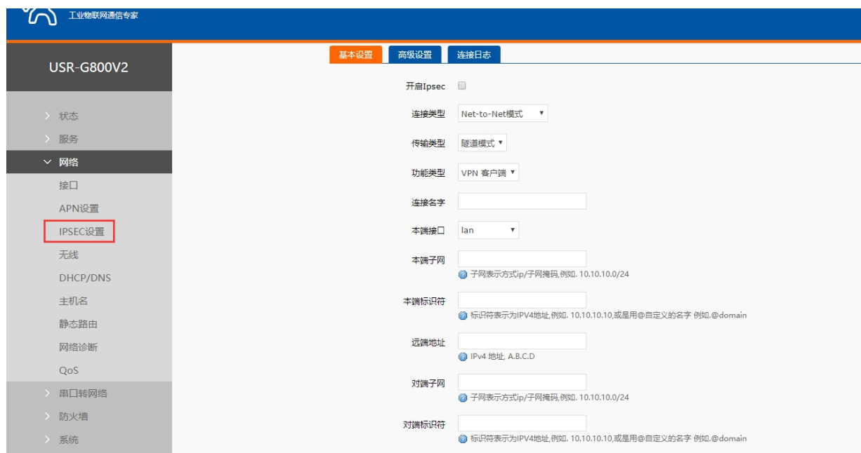
图 74 IPsec 基本设置
