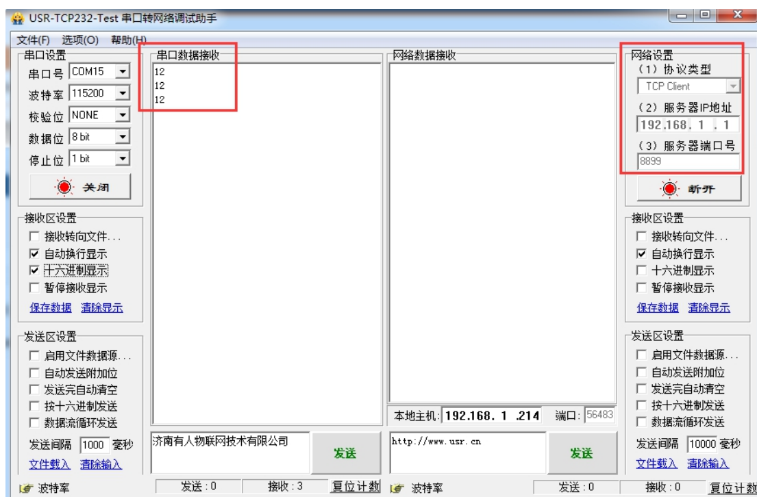
图 133 串口接收数据
