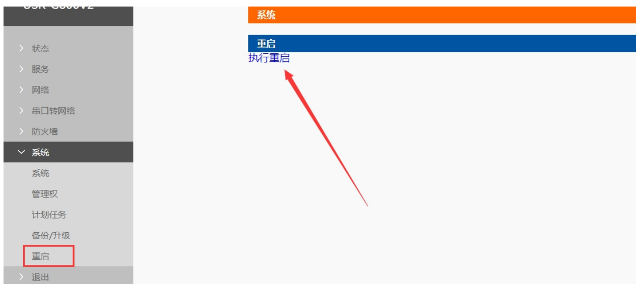
图 14 重启页面
