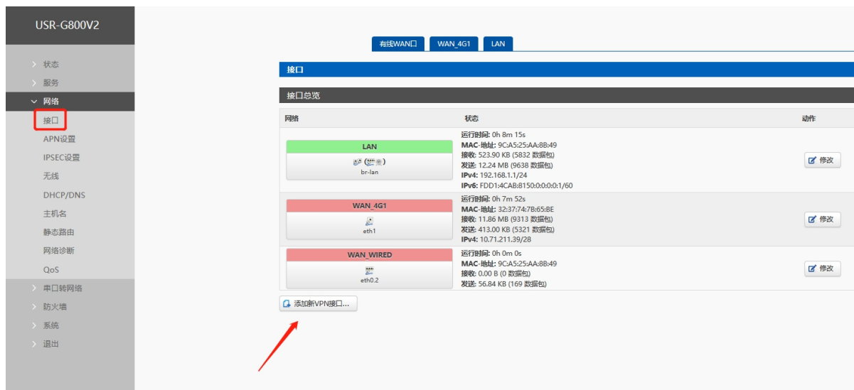
图 90 创建接口
