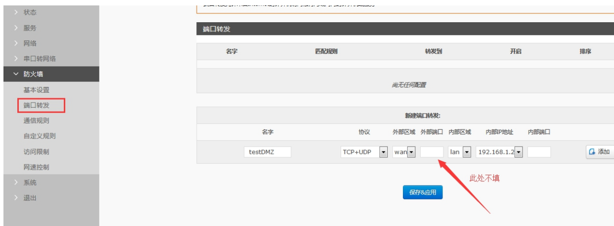
图 125 DMZ 设置一
