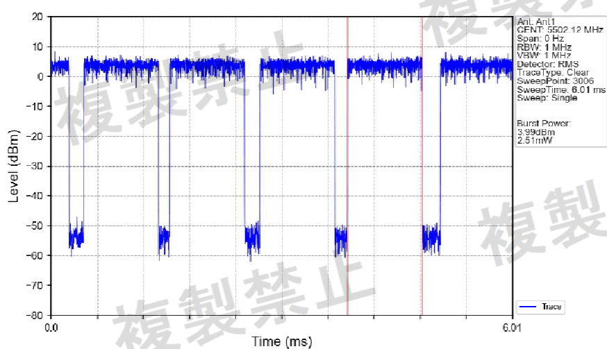
802.11ac(VHT20)_LCH_5500MHz_Ant1_NTNV
