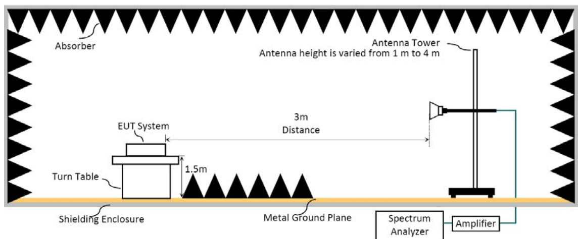
圖 2: 量測頻率高於 1GHz 之測試配置 (Fully Anechoic Chamber)
