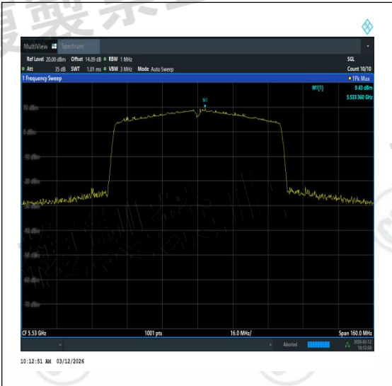
NTNV-11AC80SISO-Ant1-5530-TPC_H-PASS
