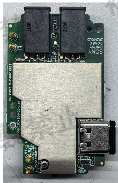
主基板(アンテナ実装面)
