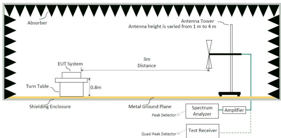
圖 1: 量測場地(3m Semi Anechoic Chamber)量測頻率低於 1GHz 之測試配置
