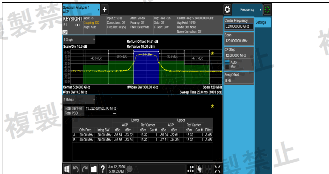
NTNV_11A_Ant1_5240
