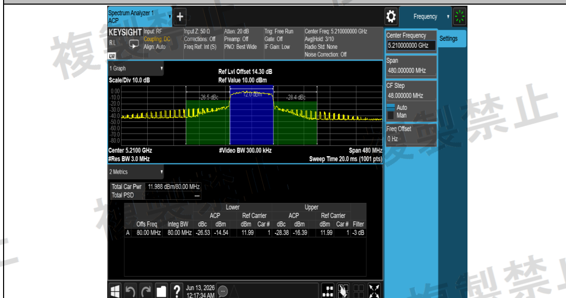
NTNV_11AC80SISO_Ant1_5210
