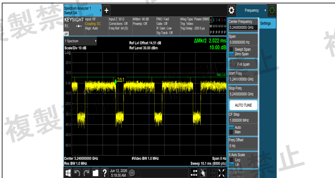
NTNV_11A_Ant1_5240
