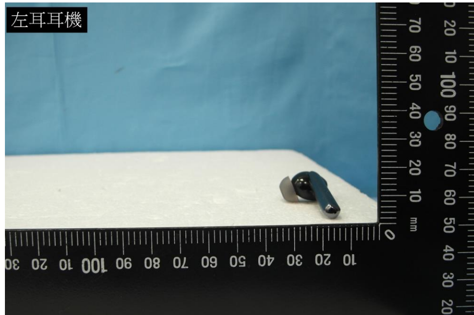
EUT Photo (10)
