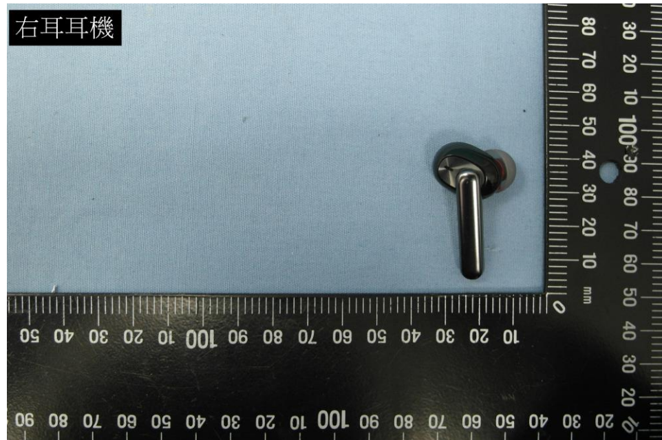
EUT Photo (12)
