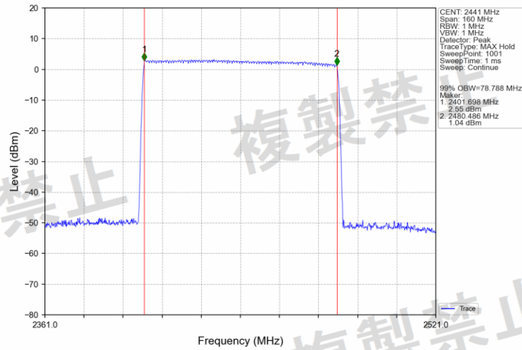
8DPSK_3DH5_HOPP_Ant1_NTLV
