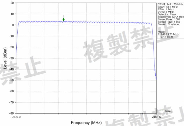
Pi/4DQPSK_2DH5_HOPP_Ant1_NTNV
