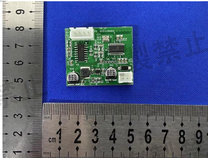
Bluetooth module
