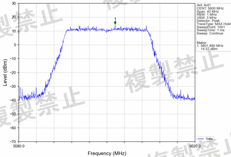
802.11be(EHT20)_MCH_5600MHz_RU242_Left_Ant1_NTNV
