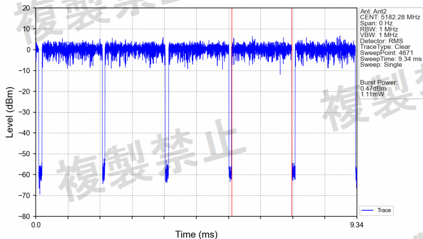
802.11be(EHT20)_LCH_5180MHz_RU242_Left_Ant2_NTNV
