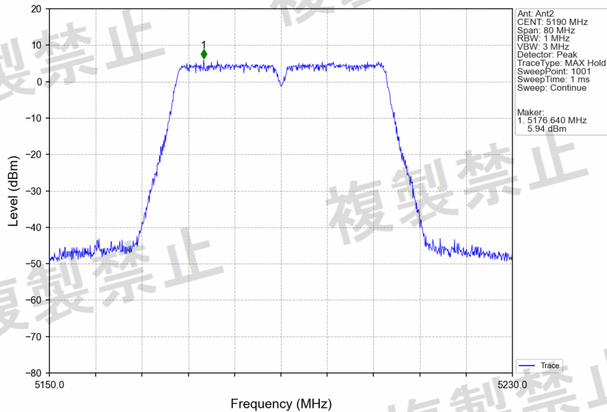
802.11n(HT40)_LCH_5190MHz_Ant2_NTNV
