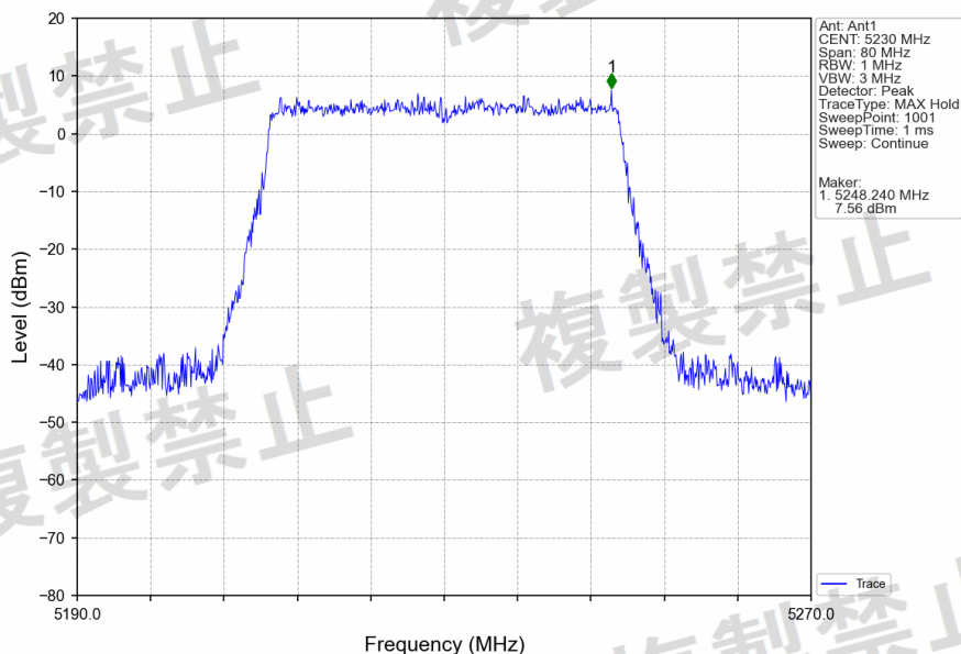
802.11be(EHT40)_HCH_5230MHz_RU484_Left_Ant1_NTNV
