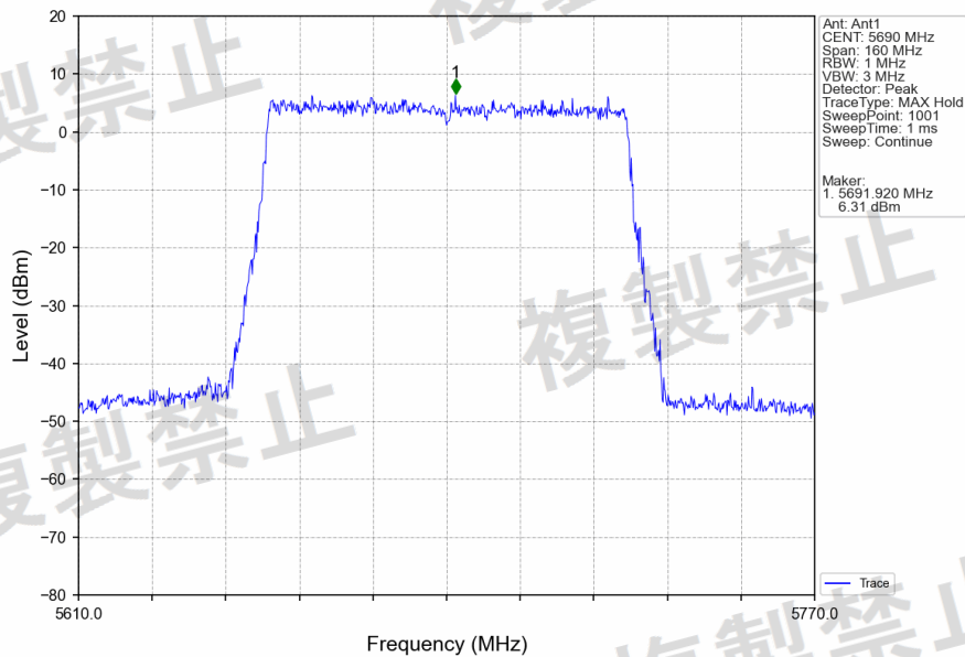
802.11ax(HEW80)_HHCH_5690MHz_RU996_Left_Ant1_NTNV
