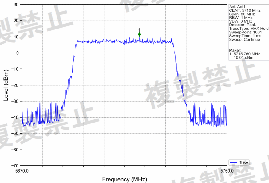
802.11ax(HEW40)_HHCH_5710MHz_RU484_Left_Ant1_NTNV
