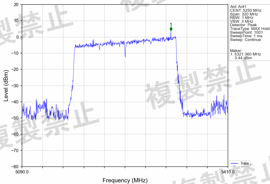
802.11ax(HEW160)_MCH_5250MHz_2xRU996_Left_Ant1_NTNV
