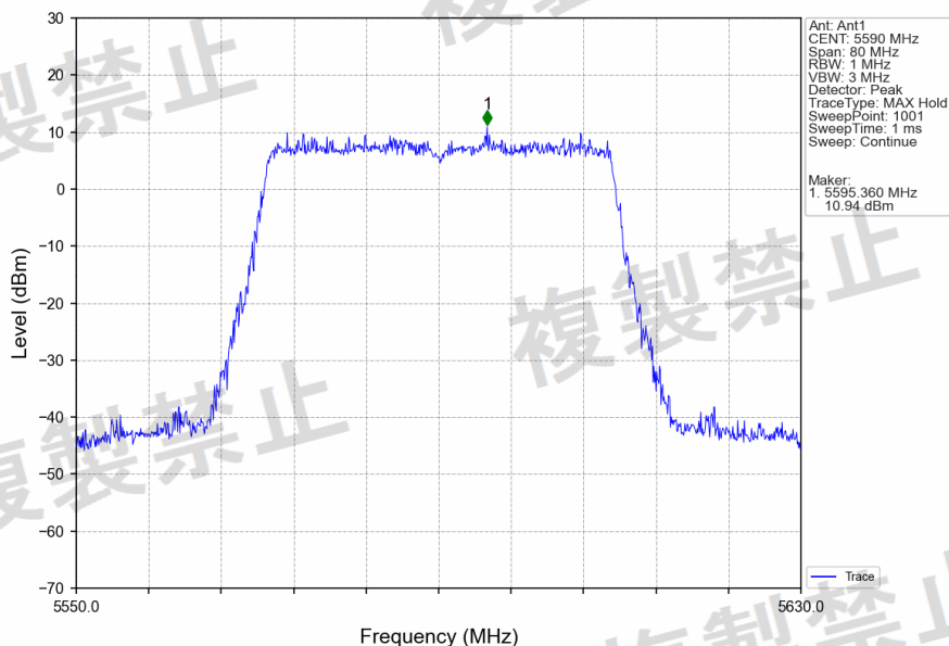
802.11be(EHT40)_MCH_5590MHz_RU484_Left_Ant1_NTNV
