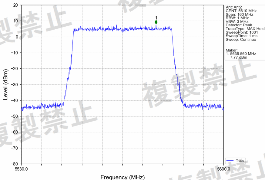
802.11ax(HEW80)_HCH_5610MHz_RU996_Left_Ant2_NTNV
