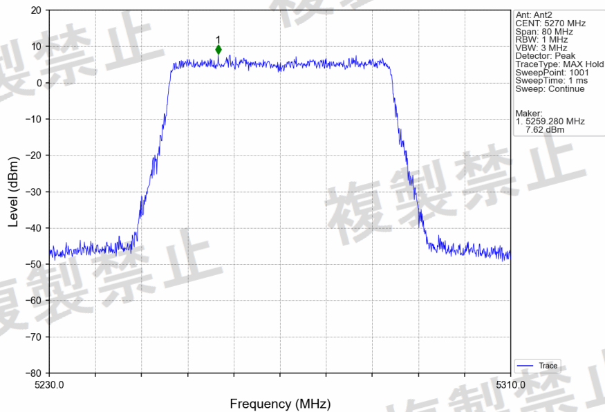
802.11ax(HEW40)_LCH_5270MHz_RU484_Left_Ant2_NTNV
