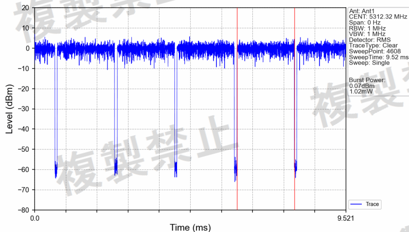
802.11be(EHT20)_HCH_5320MHz_RU242_Left_Ant1_NTNV
