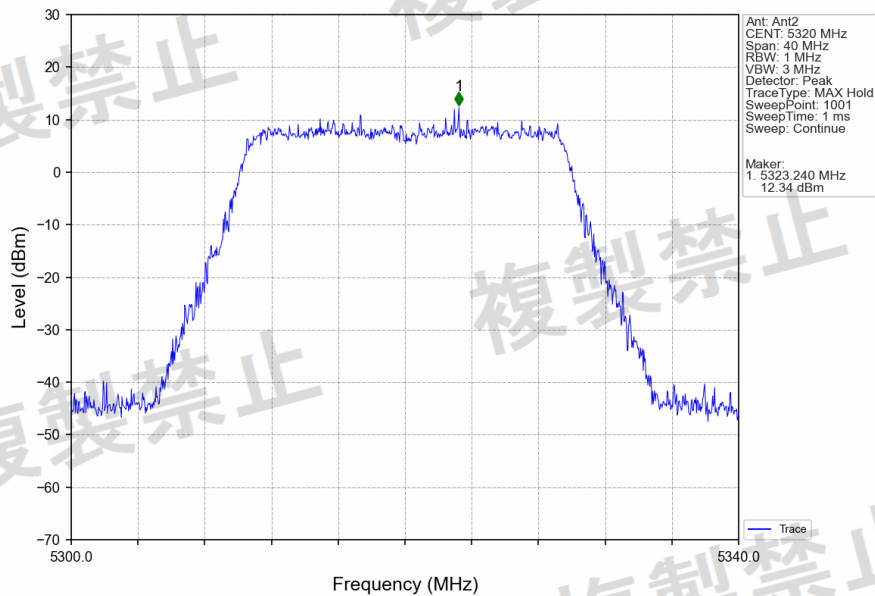
802.11ax(HEW20)_HCH_5320MHz_RU242_Left_Ant2_NTNV
