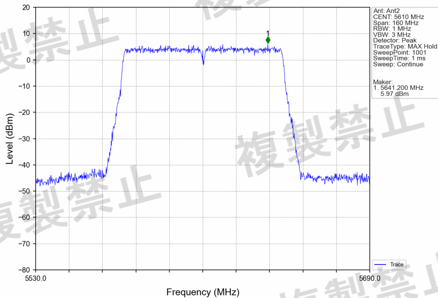
802.11ac(VHT80)_HCH_5610MHz_Ant2_NTNV
