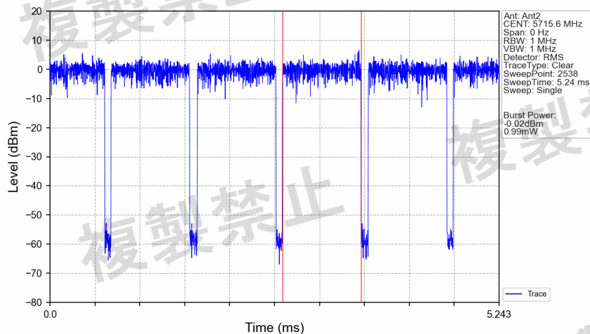
802.11be(EHT40)_HHCH_5710MHz_RU484_Left_Ant2_NTNV
