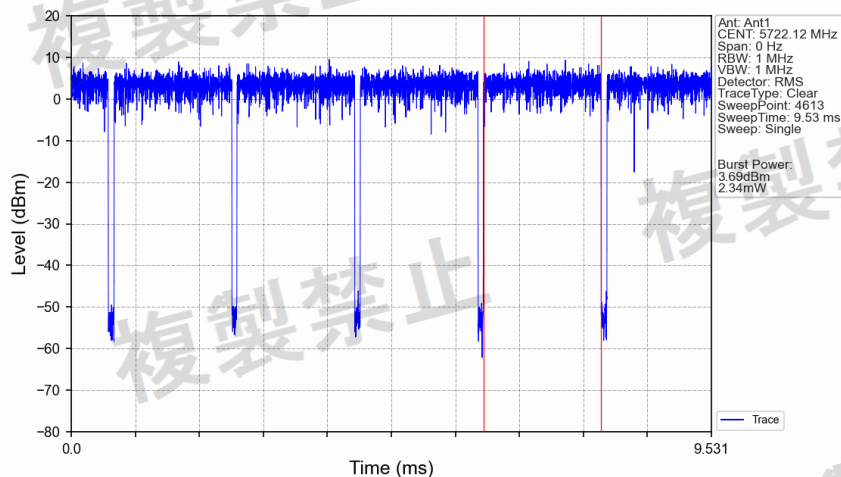
802.11be(EHT20)_HHCH_5720MHz_RU242_Left_Ant1_NTNV
