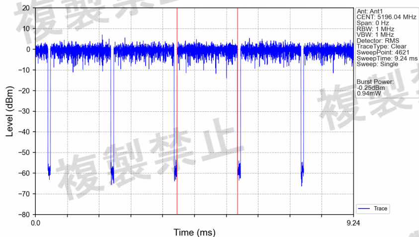
802.11be(EHT20)_MCH_5200MHz_RU242_Left_Ant1_NTNV
