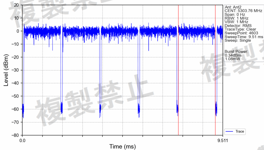
802.11be(EHT20)_MCH_5300MHz_RU242_Left_Ant2_NTNV
