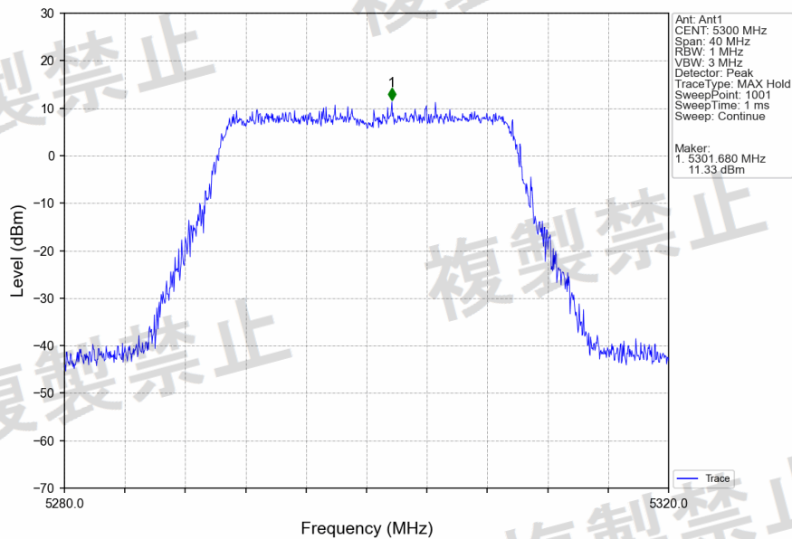
802.11be(EHT20)_MCH_5300MHz_RU242_Left_Ant1_NTNV
