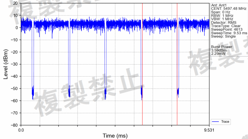
802.11be(EHT20)_LCH_5500MHz_RU242_Left_Ant1_NTNV
