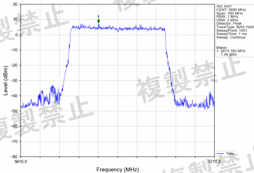
802.11be(EHT80)_HHCH_5690MHz_RU996_Left_Ant1_NTNV
