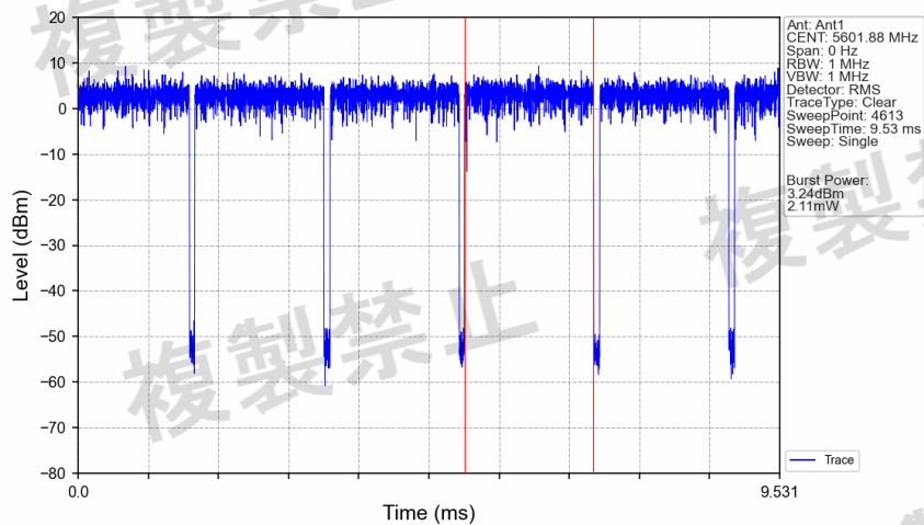
802.11be(EHT20)_MCH_5600MHz_RU242_Left_Ant1_NTNV
