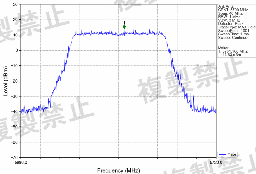
802.11be(EHT20)_HCH_5700MHz_RU242_Left_Ant2_NTNV
