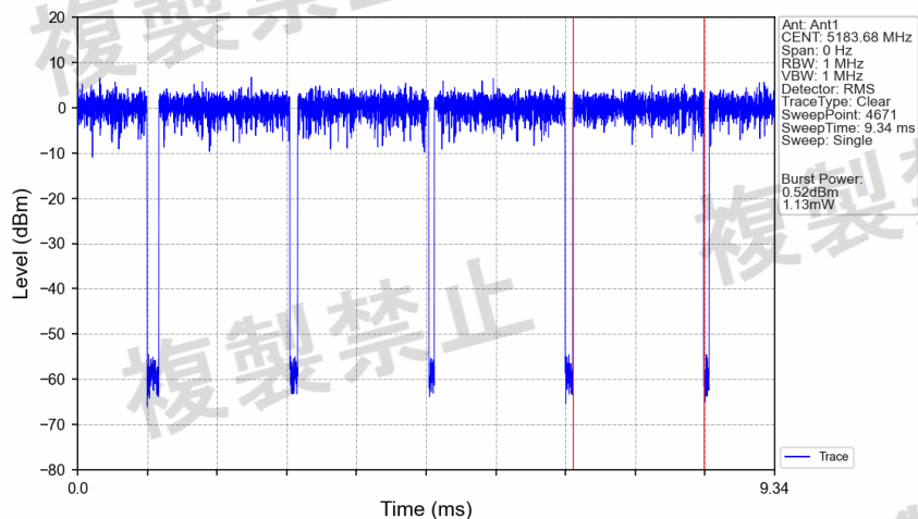
802.11be(EHT20)_LCH_5180MHz_RU242_Left_Ant1_NTNV
