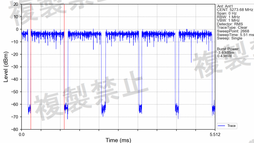
802.11ac(VHT40)_LCH_5270MHz_Ant1_NTNV
