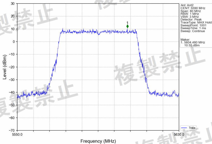
802.11be(EHT40)_MCH_5590MHz_RU484_Left_Ant2_NTNV
