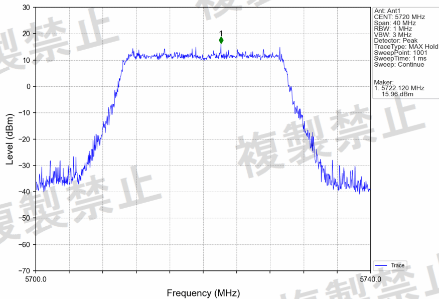
802.11be(EHT20)_HHCH_5720MHz_RU242_Left_Ant1_NTNV
