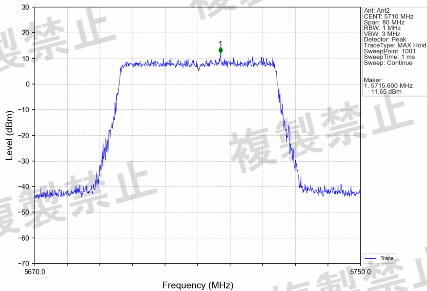
802.11be(EHT40)_HHCH_5710MHz_RU484_Left_Ant2_NTNV
