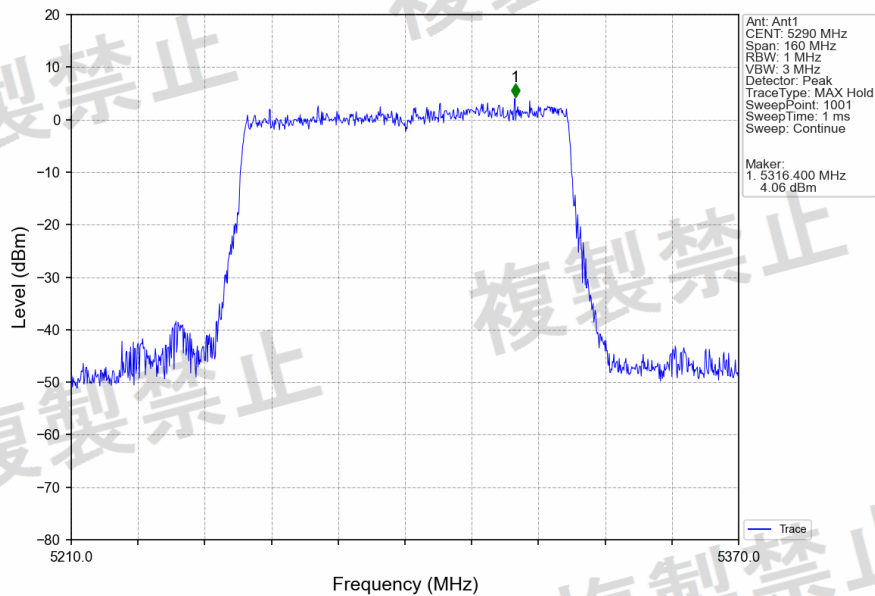
802.11be(EHT80)_MCH_5290MHz_RU996_Left_Ant1_NTNV
