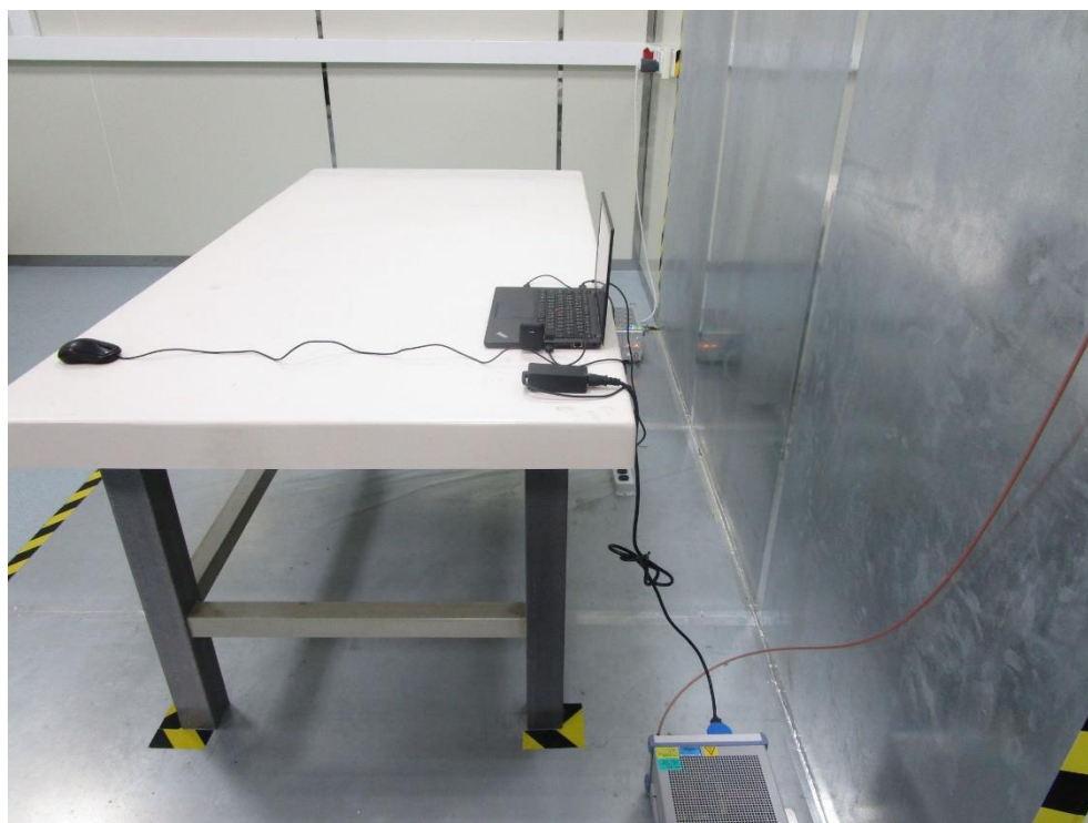
測試模式: Mode 4 電源傳導測試 側面照 - 0.15MHz ~ 30MHz
