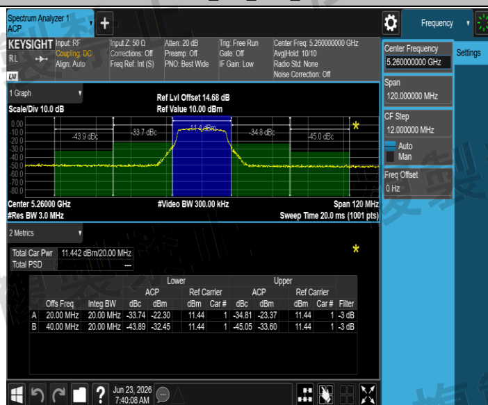
NTNV_11A_Ant1_5260
