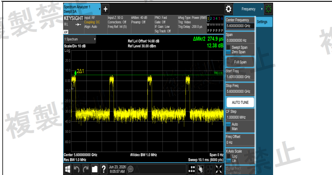
NTNV_11A_Ant1_5600
