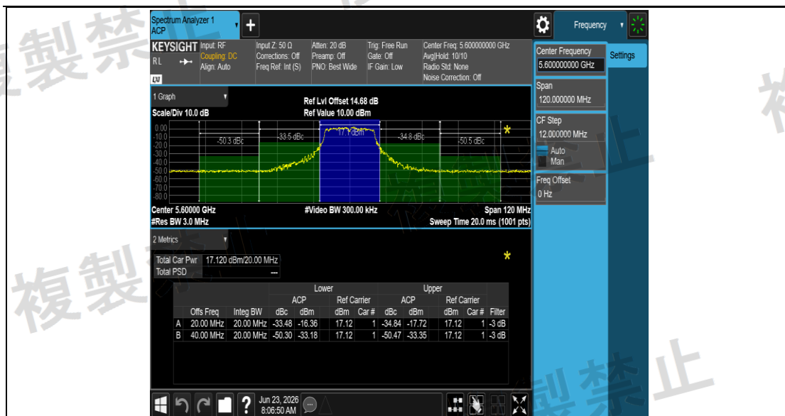
NTNV_11A_Ant1_5600
