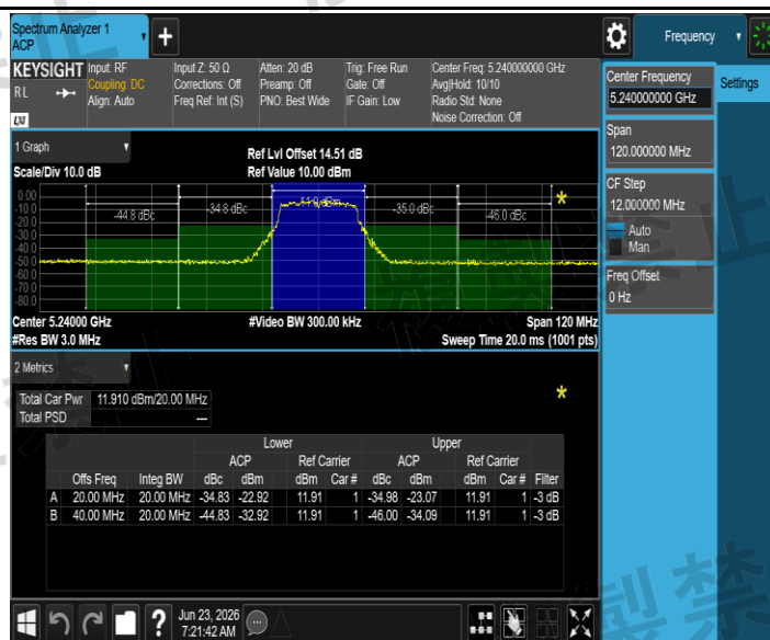
NTNV_11A_Ant1_5240
