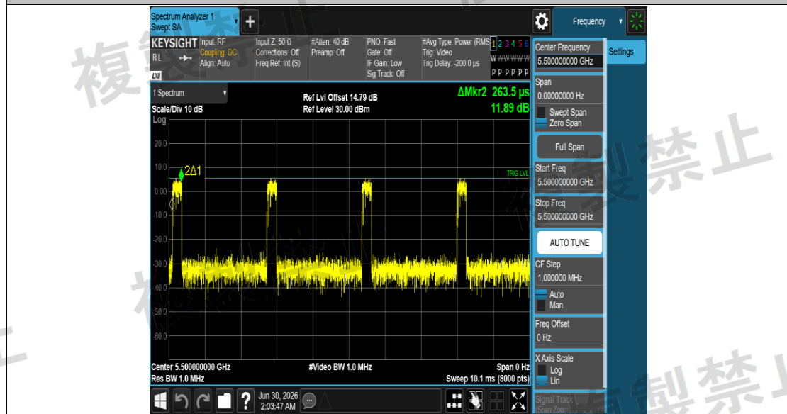
NTNV_11AX20SISO_Ant1_5500
