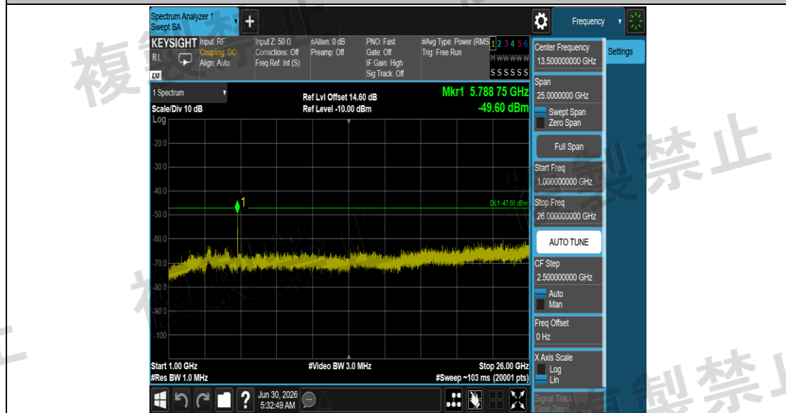
NTNV_11A_Ant1_5720_1000~26000
