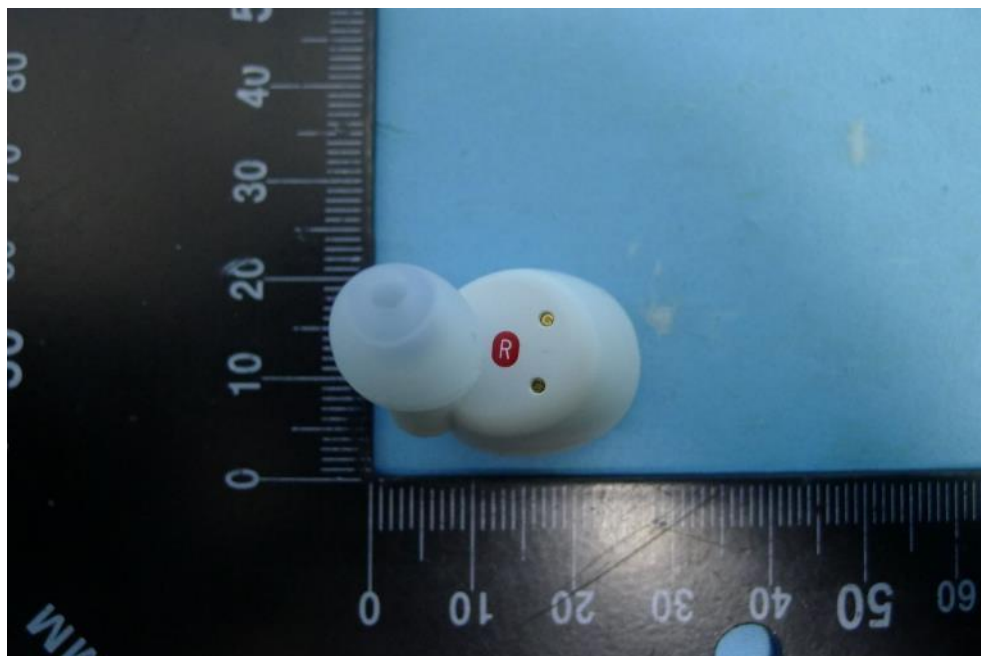
(8) 待測物照片 (右耳 白)
