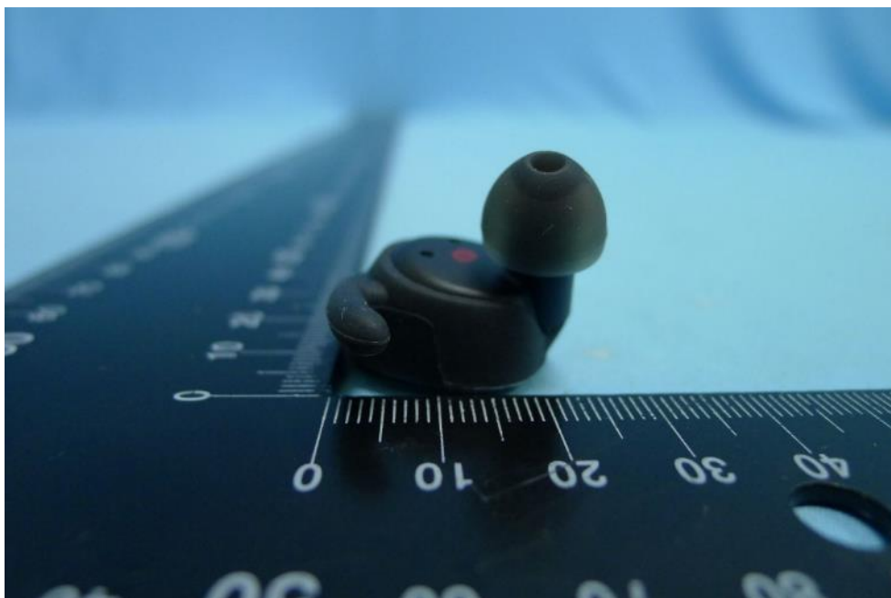
(5) 待測物照片 (右耳 黑)
