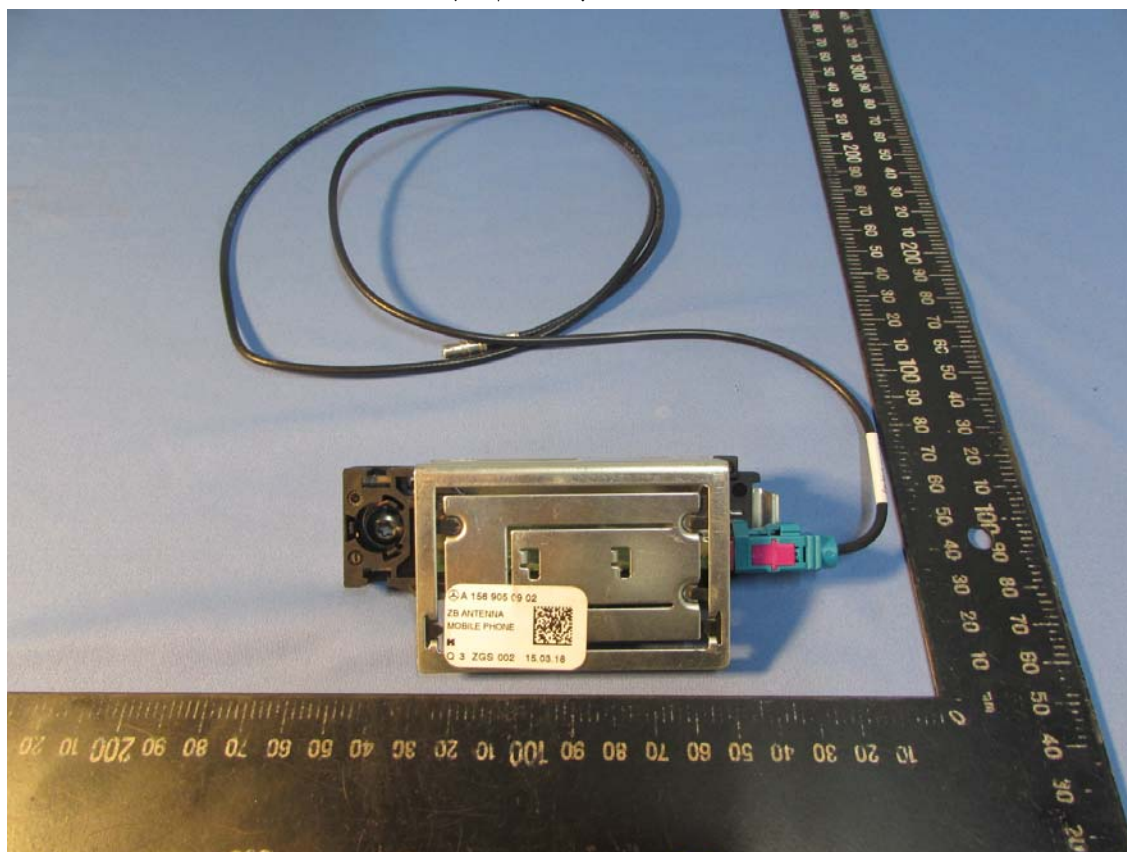
外部天線2 正面照
