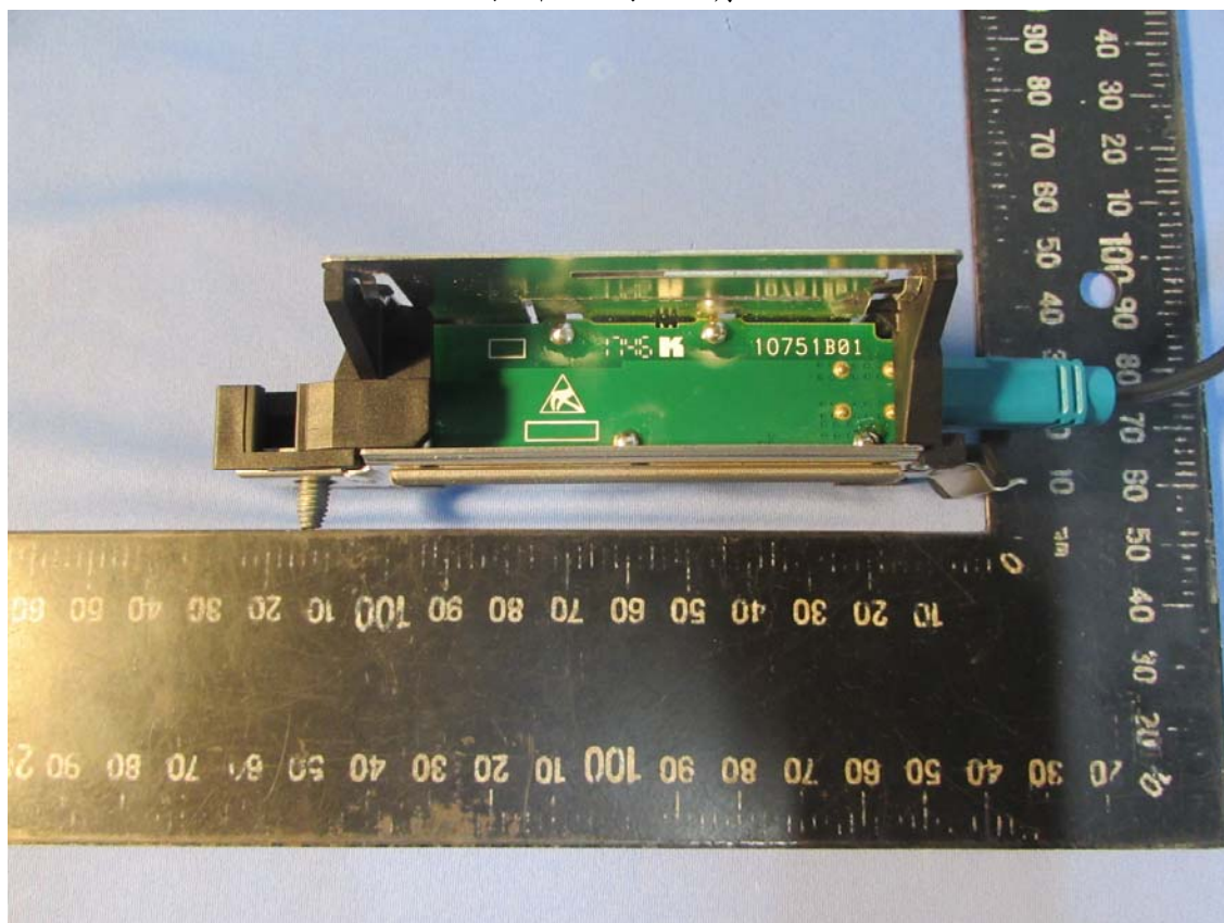
外部天線2 背面照
