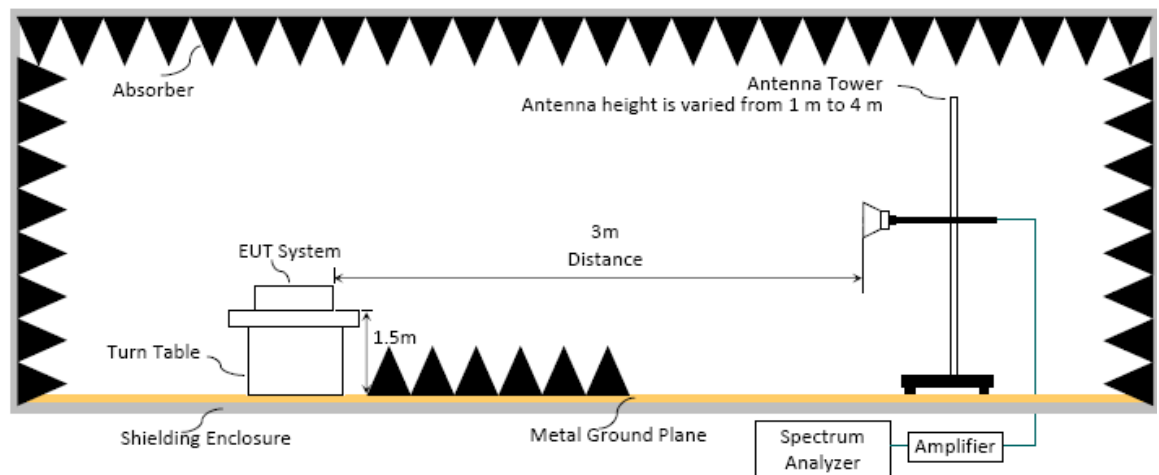
圖 2: 量測頻率高於 1GHz 之測試配置 (3m Semi Anechoic Chamber)
