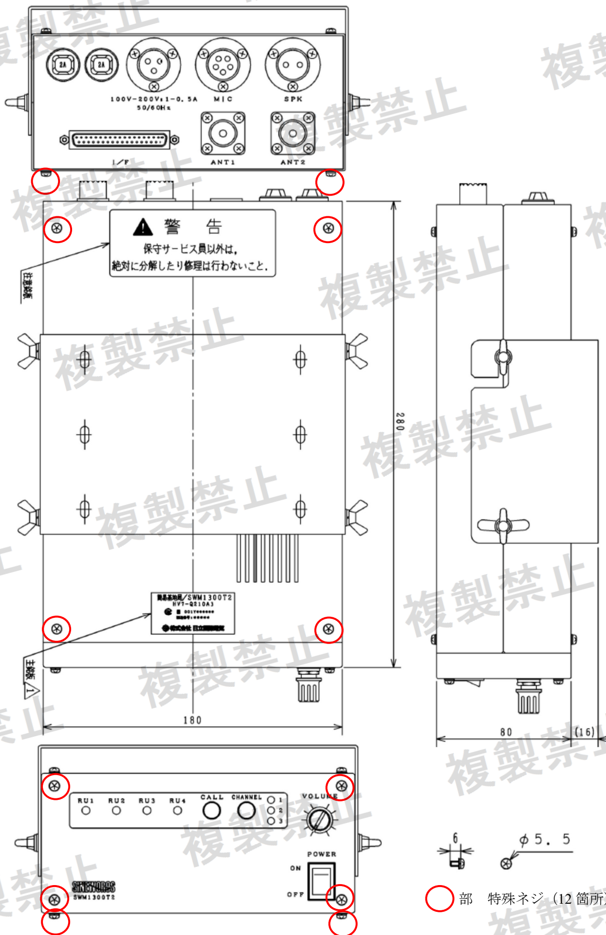
機器外觀図
