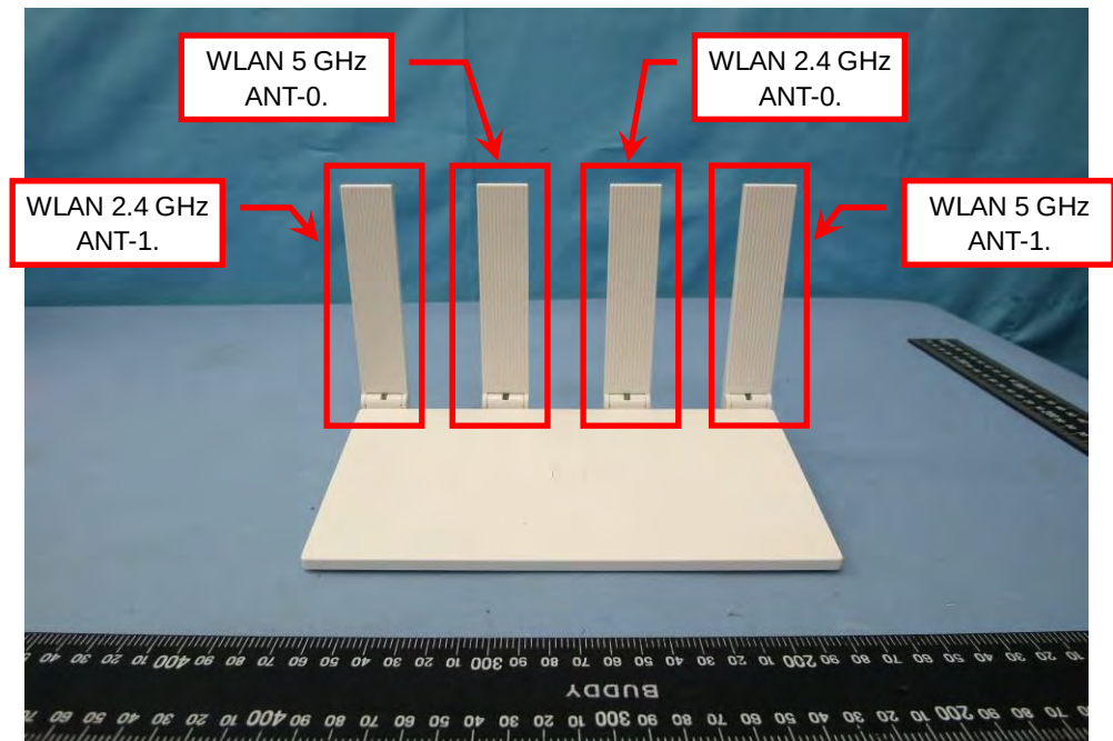
EUT Photo (6)
