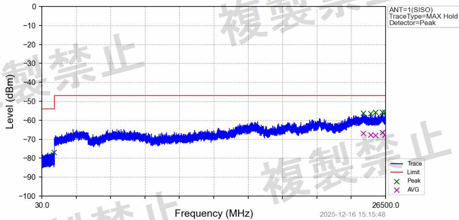
802.11ac(VHT40) LCH_5190MHz_Ant1_NTNV
