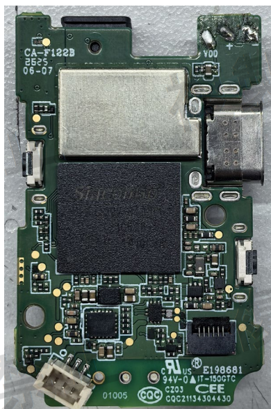
主基板
