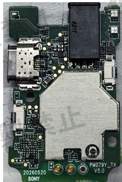
主基板(アンテナ実装面)
