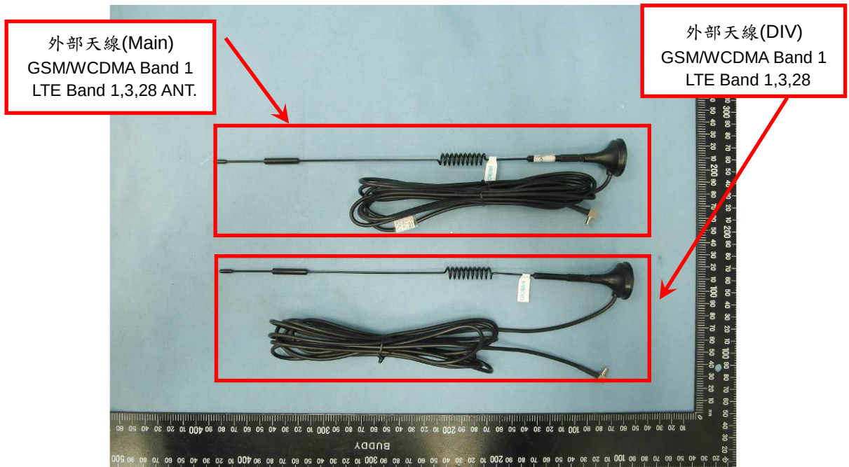
EUT Photo (12)
