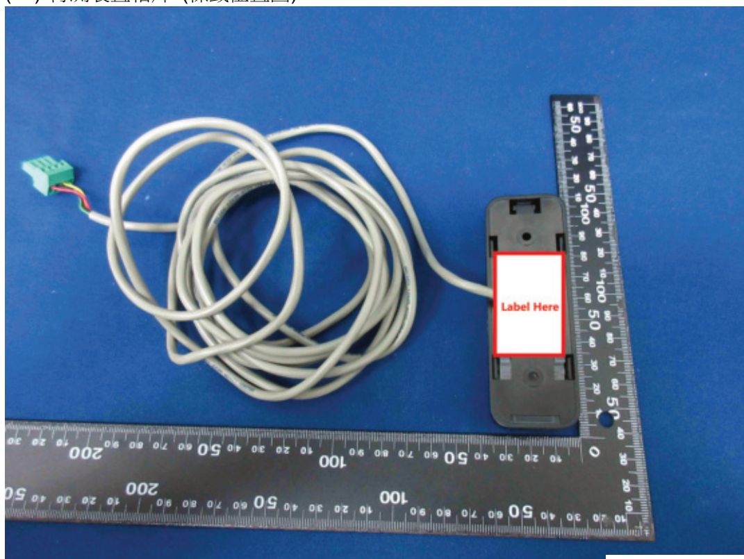
(28) 待測裝置相片 (標籤位置圖)
