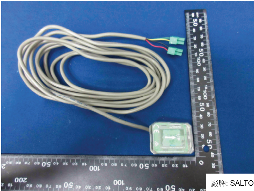
(2) 待測裝置相片
