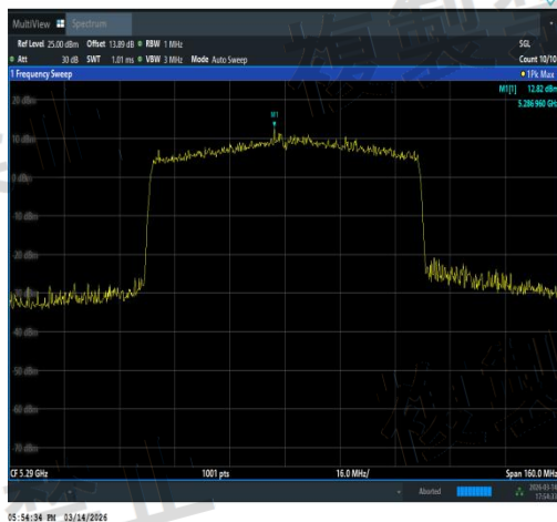
NTNV-11AX80SISO-Ant2-5290-TPC_H-PASS
