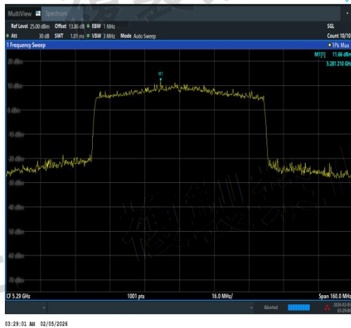
NTNV-11AX80SISO-Ant1-5290-TPC_H-PASS
