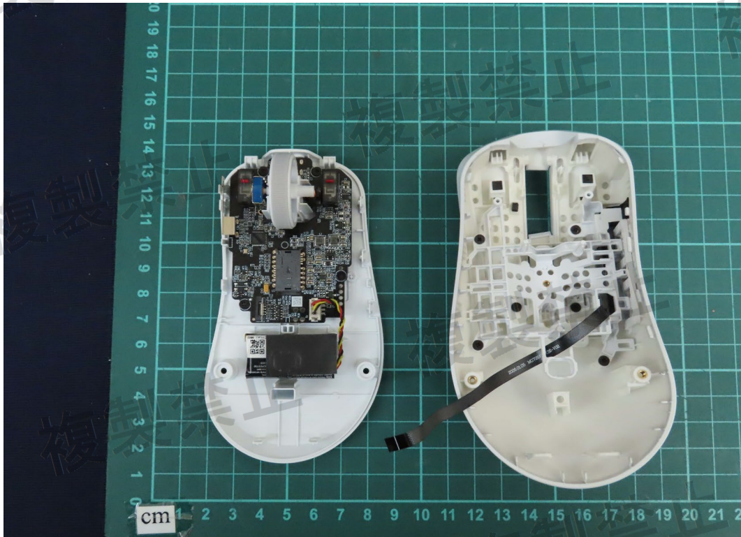
(14) EUT Photo
