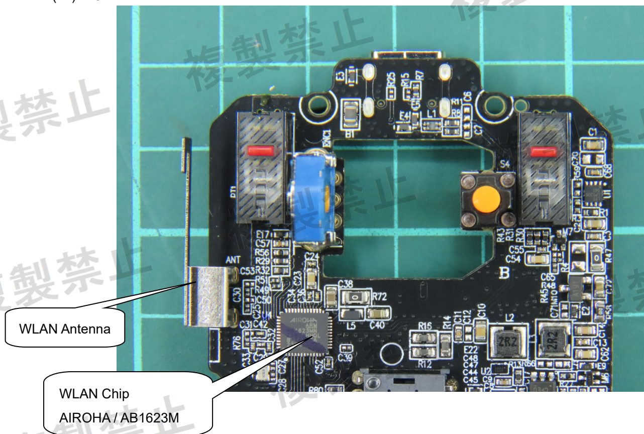
(24) EUT Photo
