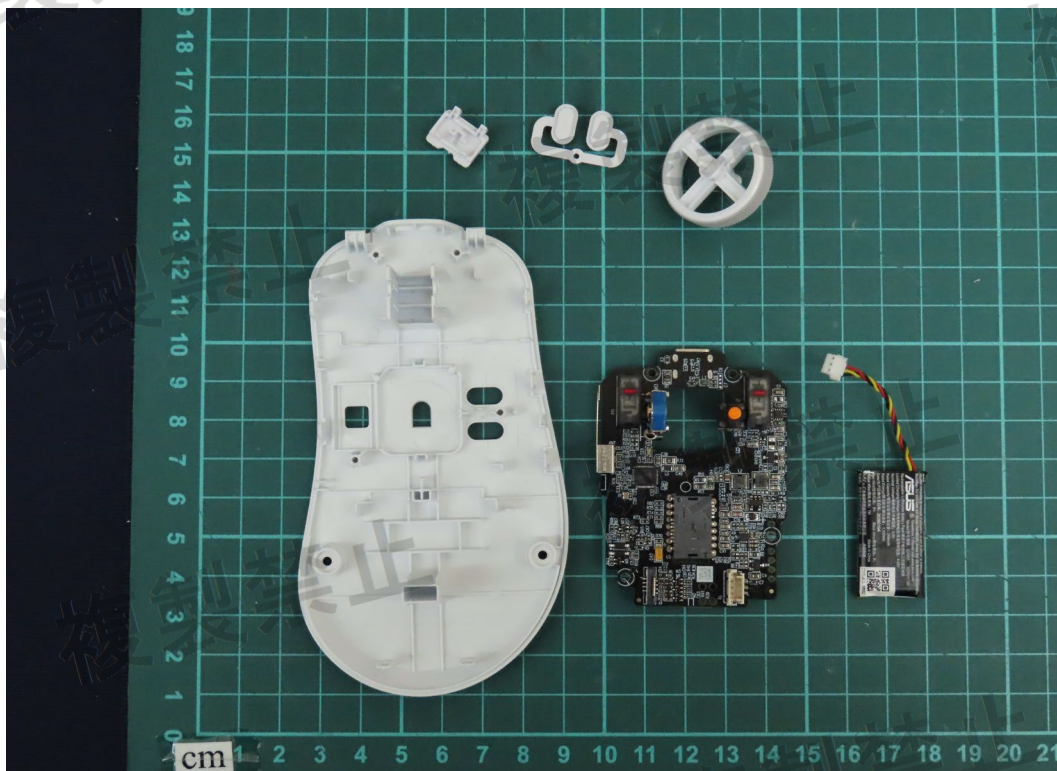
(20) EUT Photo
