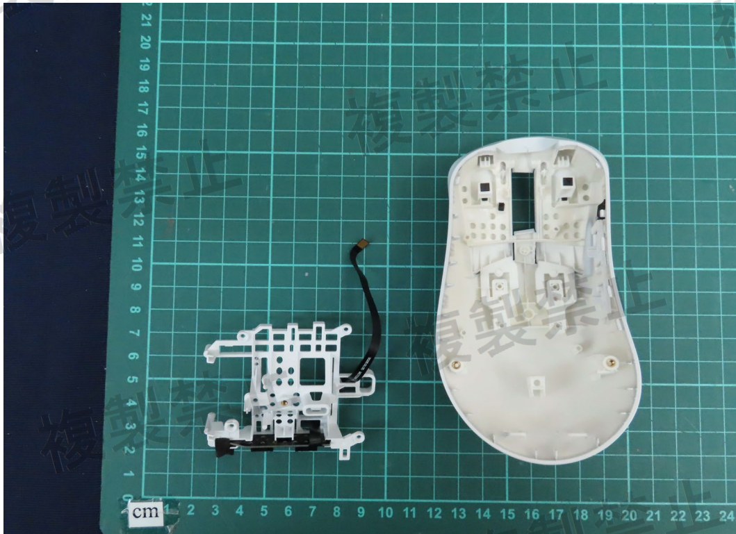
(16) EUT Photo
