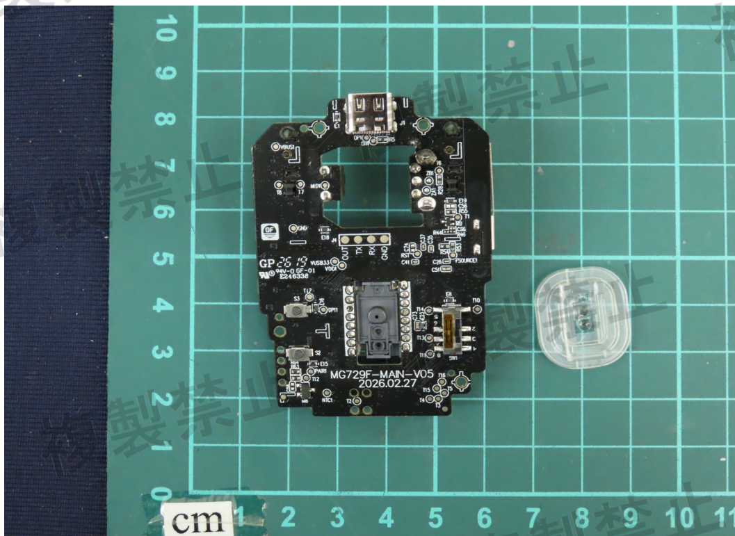
(30) EUT Photo
