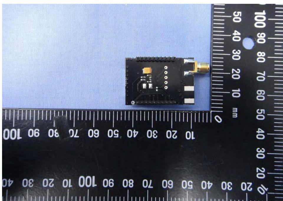
EUT Photo 4 )
