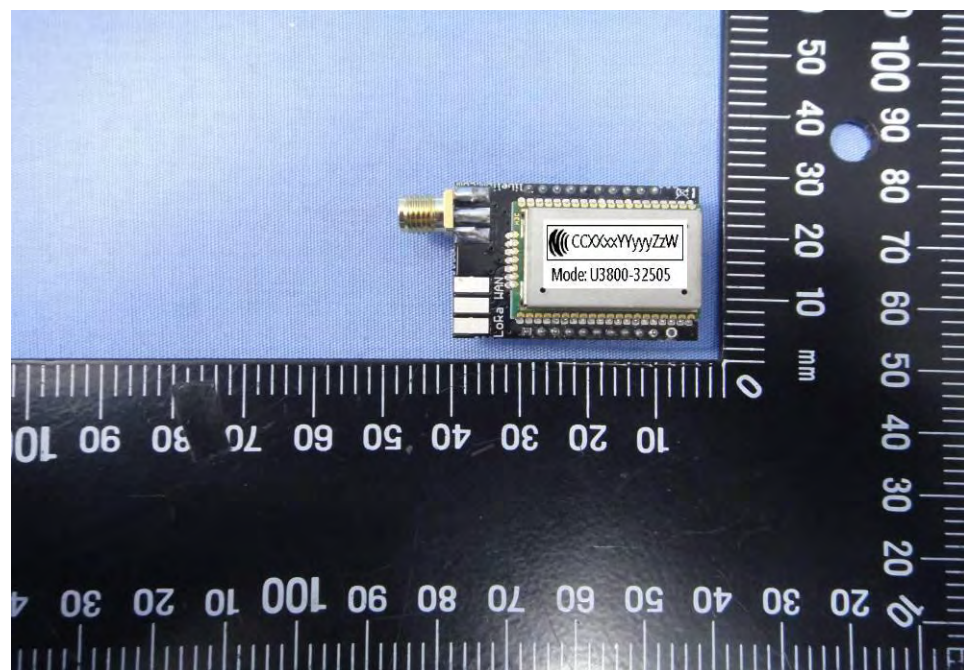
EUT Photo 2 )
