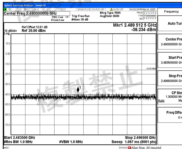
NTNV_DH5_Ant1_2402_2483.5~2496.5
