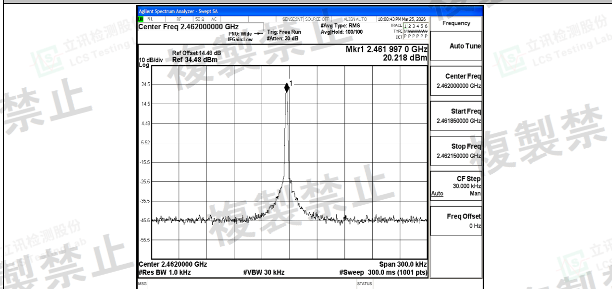
NTNV_Ant1_2462
