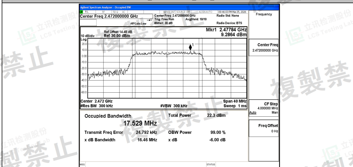
NTNV_11AX20SISO_Ant1_2472
