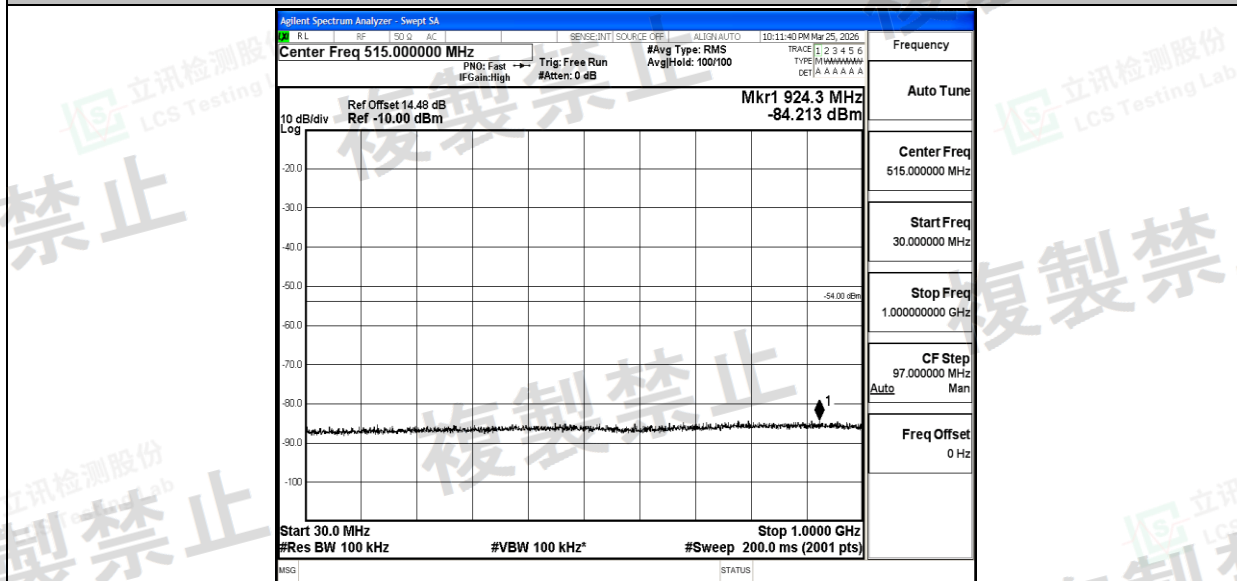
NTNV_11B_Ant1_2472_30~1000
