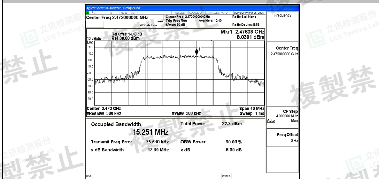
NTNV_11AX20SISO_Ant1_2472
