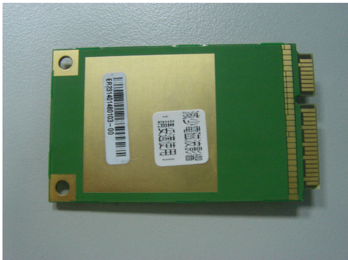
AirPrime MC7355 背面照
