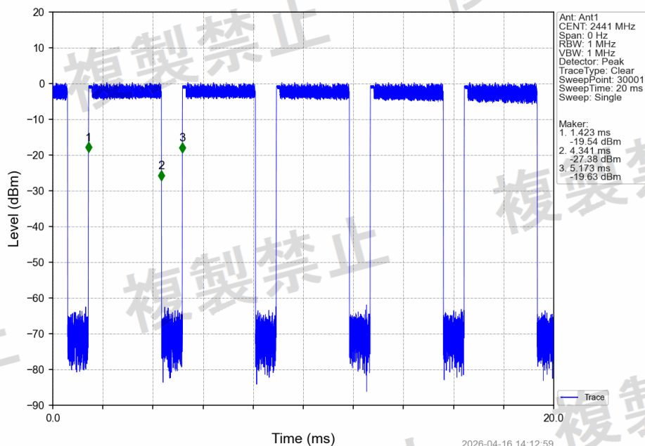
8DPSK 3DH5 2441MHz Ant1 NTLV
