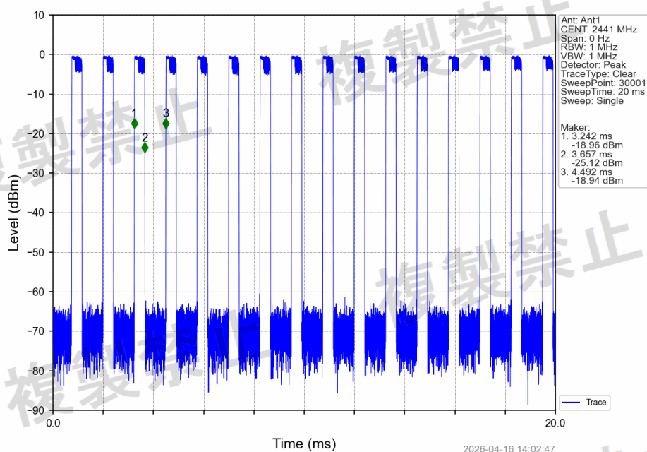
Pi/4DQPSK 2DH3 2441MHz Ant1 NTLV
