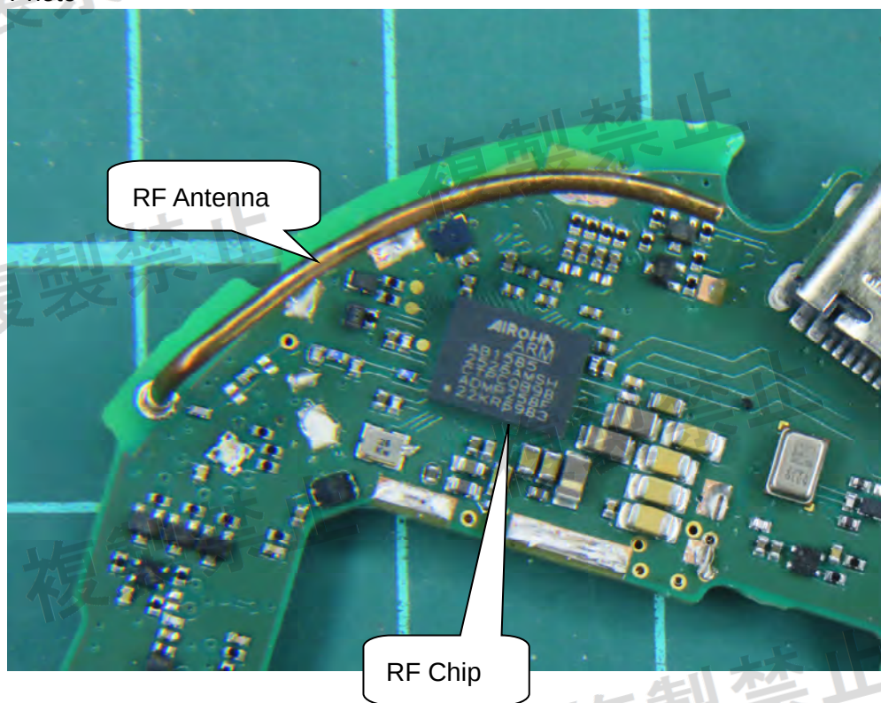
(15) EUT Photo
